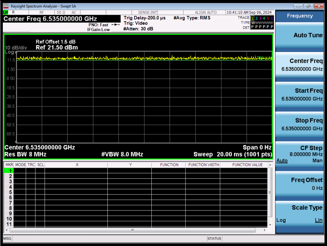
NTNV-11BE20SISO-Ant1-6535
