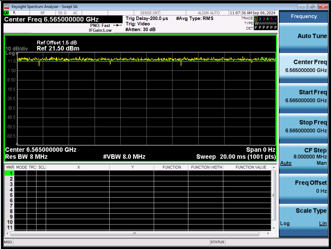
NTNV-11BE40SISO-Ant1-6565
