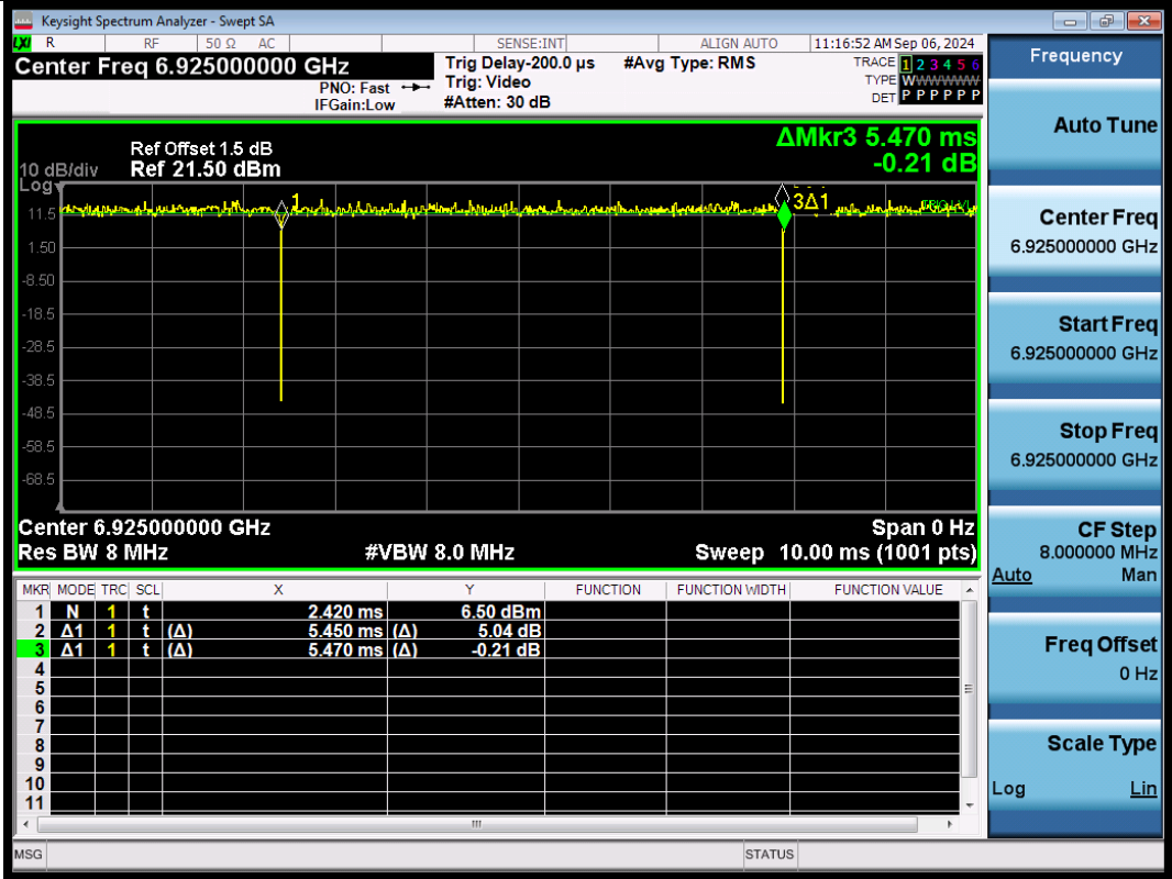
NTNV-11BE40SISO-Ant1-6925
