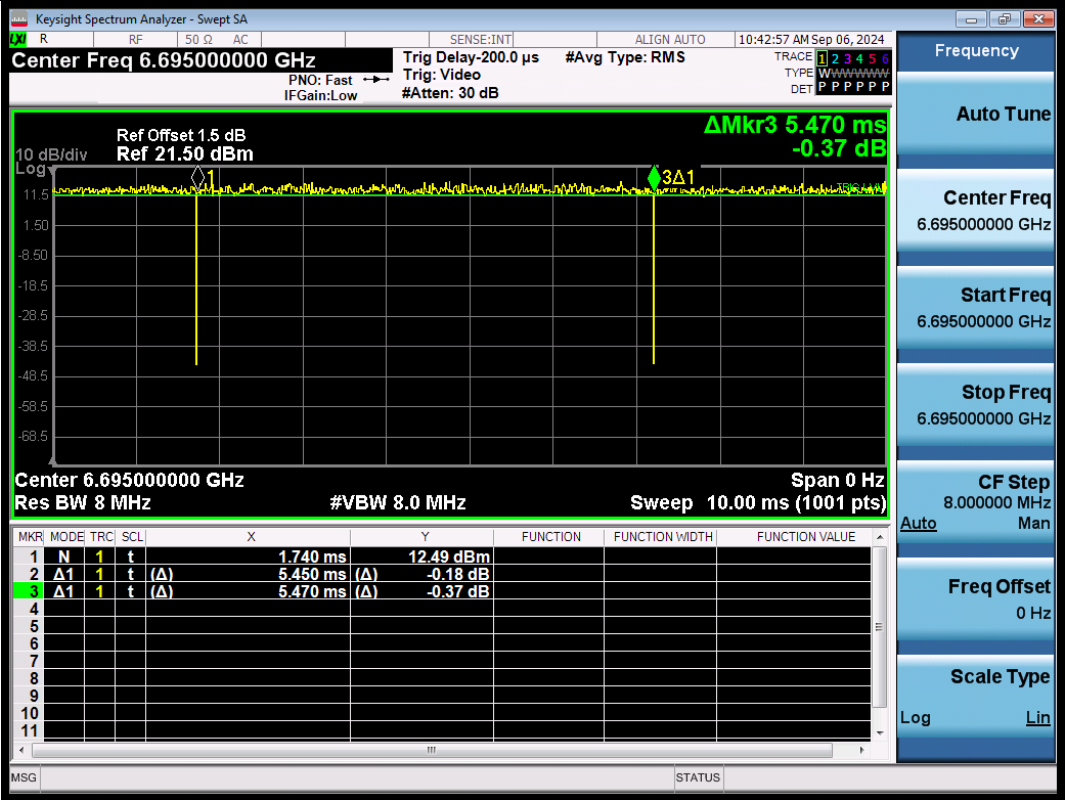
NTNV-11BE20SISO-Ant1-6695
