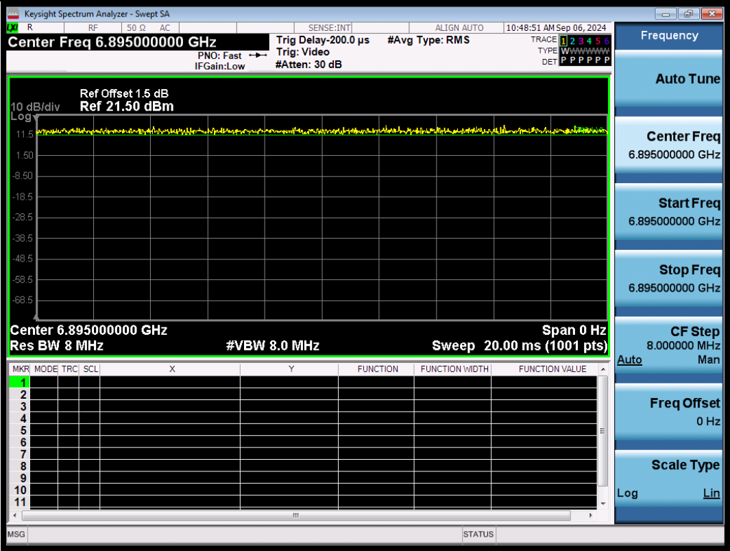
NTNV-11BE20SISO-Ant1-6895
