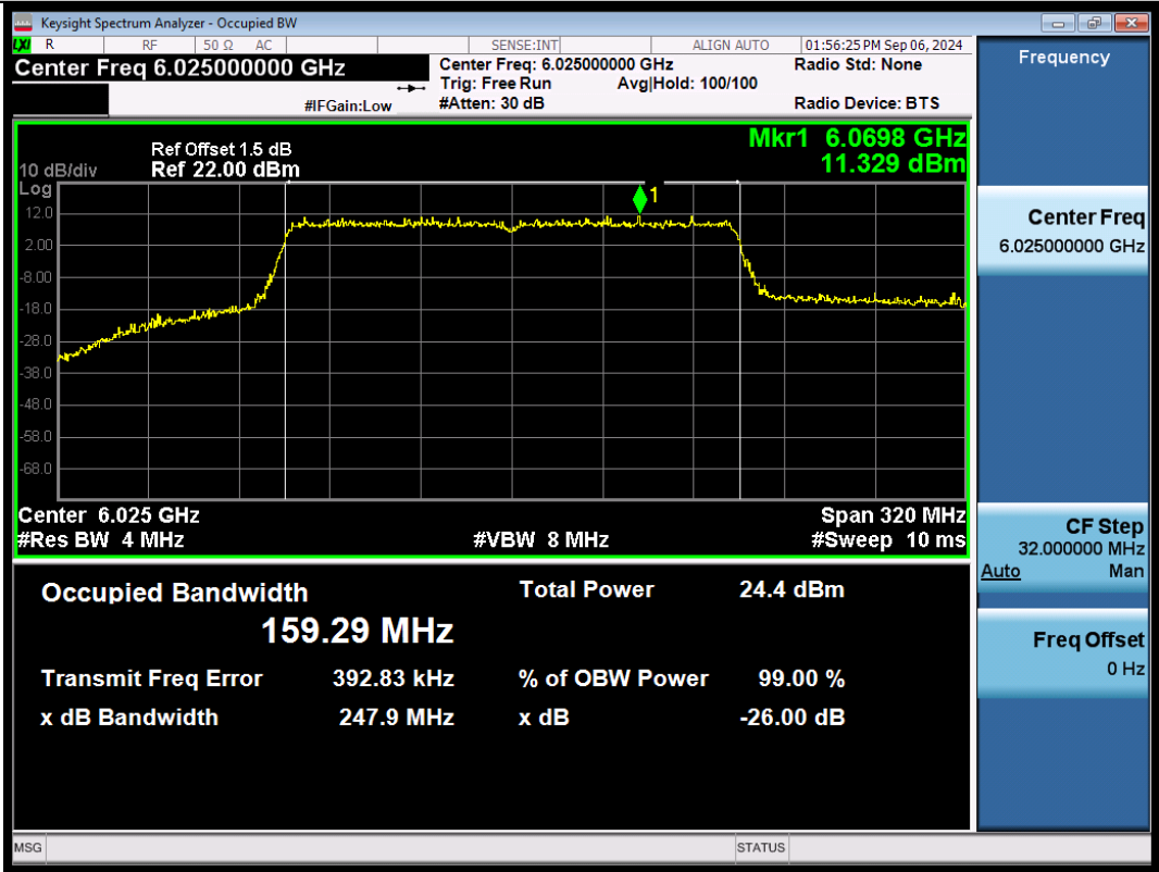
11BE160SISO-Ant1-6025-PASS
