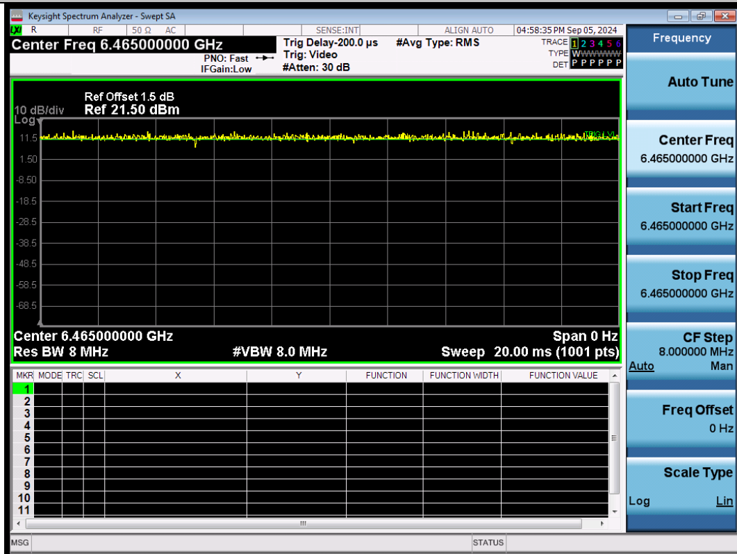
NTNV-11AX80SISO-Ant1-6465
