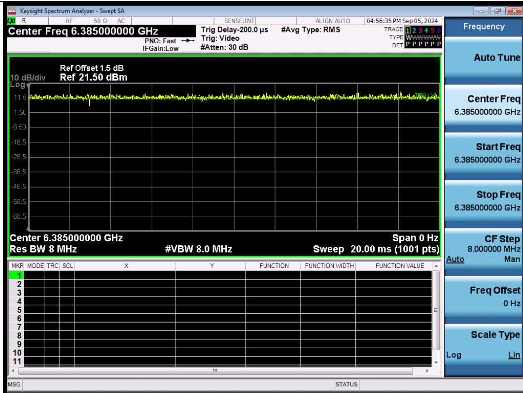
NTNV-11AX80SISO-Ant1-6385
