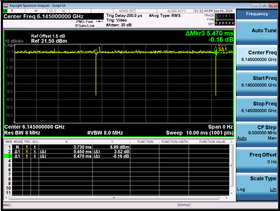
NTNV-11BE80SISO-Ant1-6145
