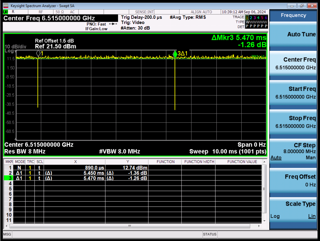
NTNV-11BE20SISO-Ant1-6515
