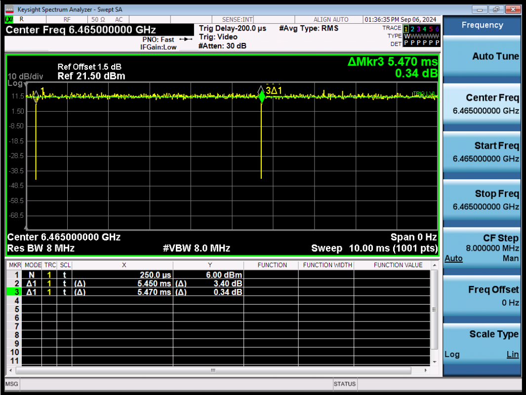
NTNV-11BE80SISO-Ant1-6465
