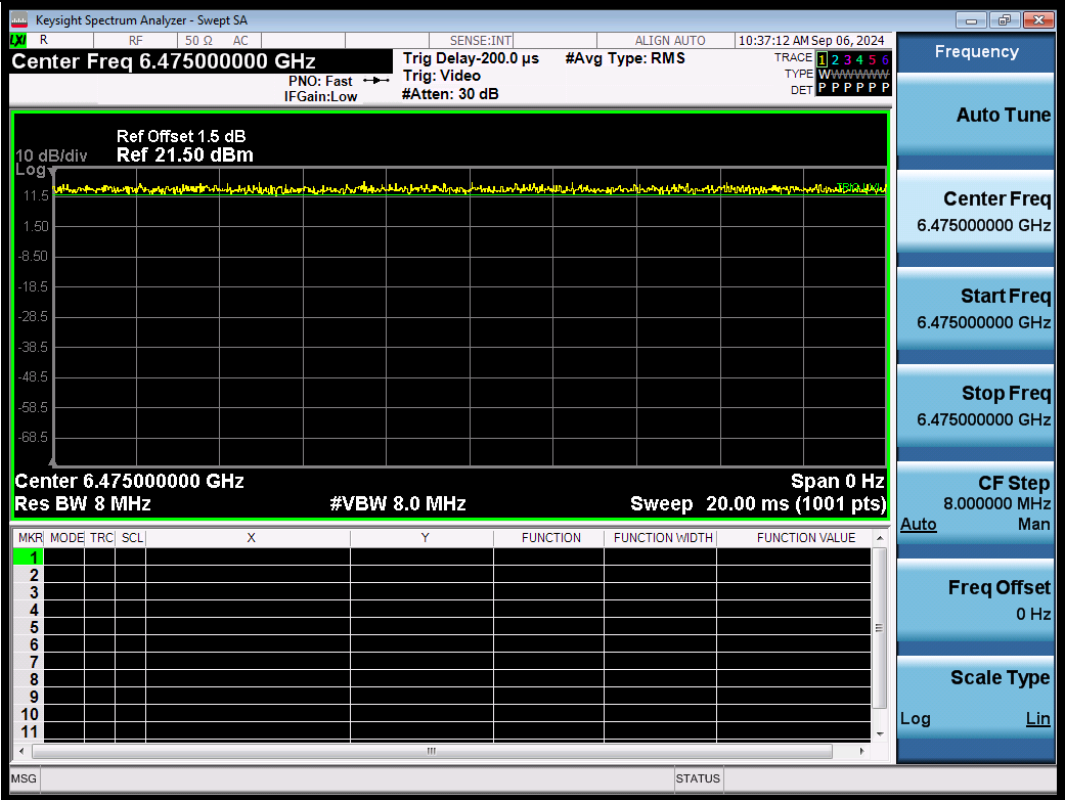
NTNV-11BE20SISO-Ant1-6475
