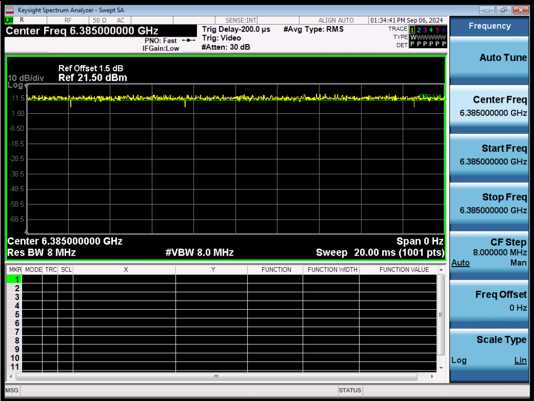
NTNV-11BE80SISO-Ant1-6385
