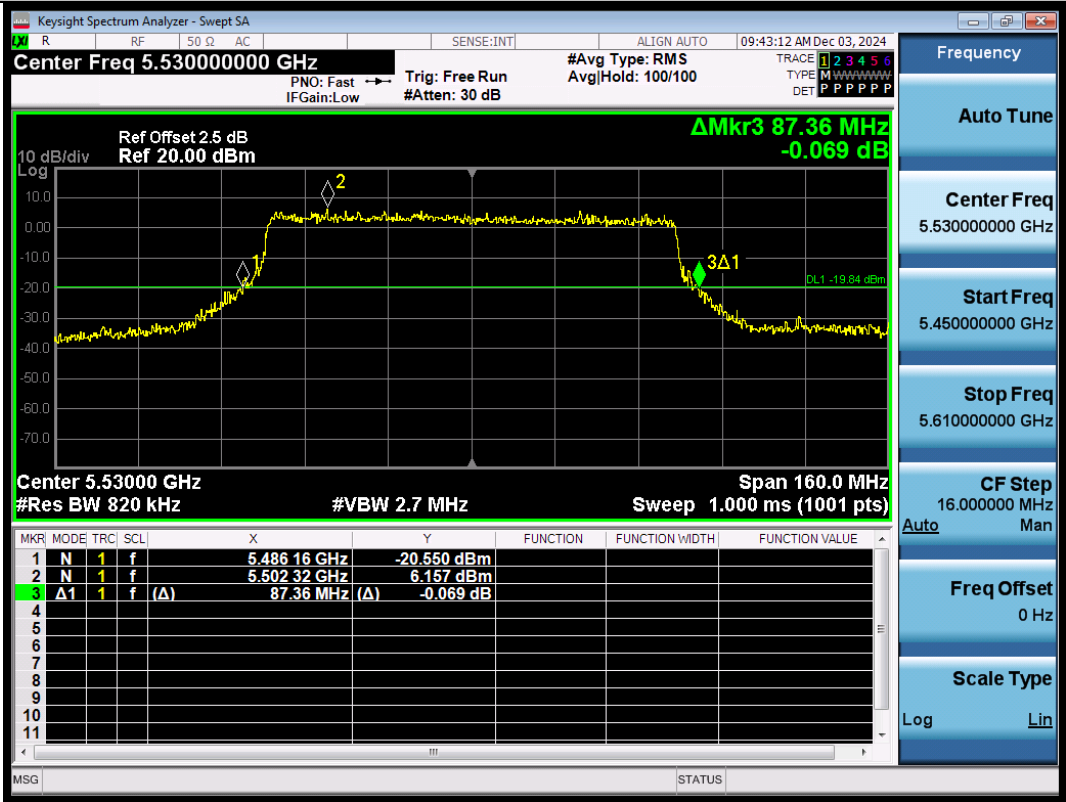
11AX80SISO-Ant3-5530
