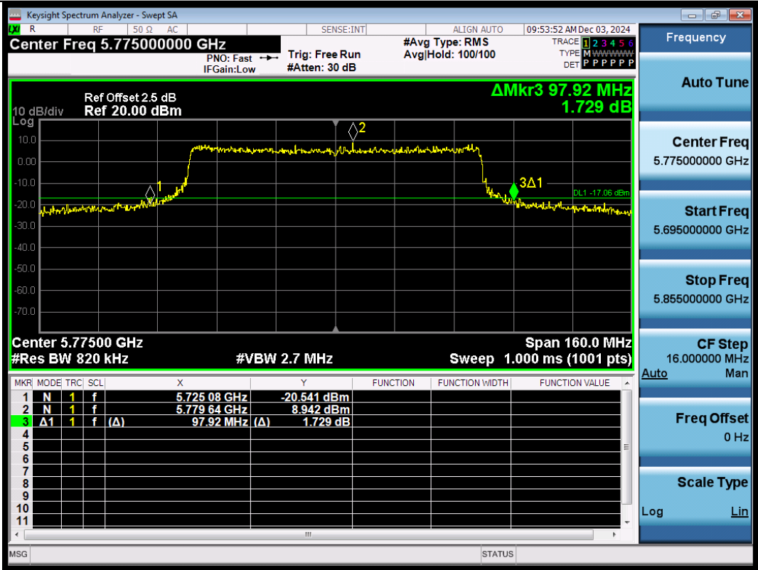
11AX80SISO-Ant3-5775
