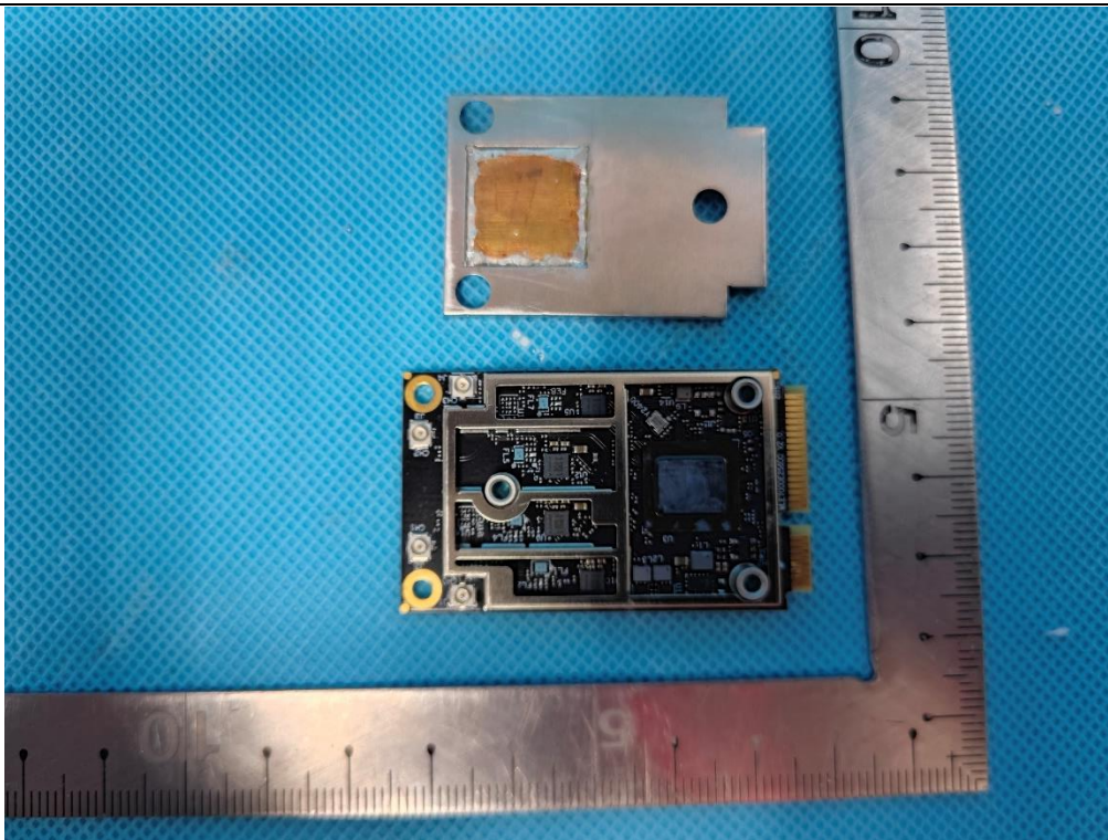
EUT Photo(6) - WLE7000E5
