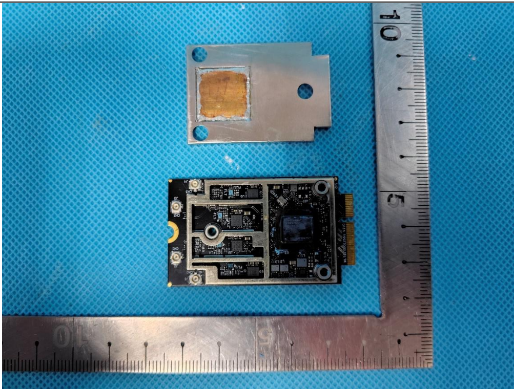
EUT Photo(10) - WLTE7000E5
