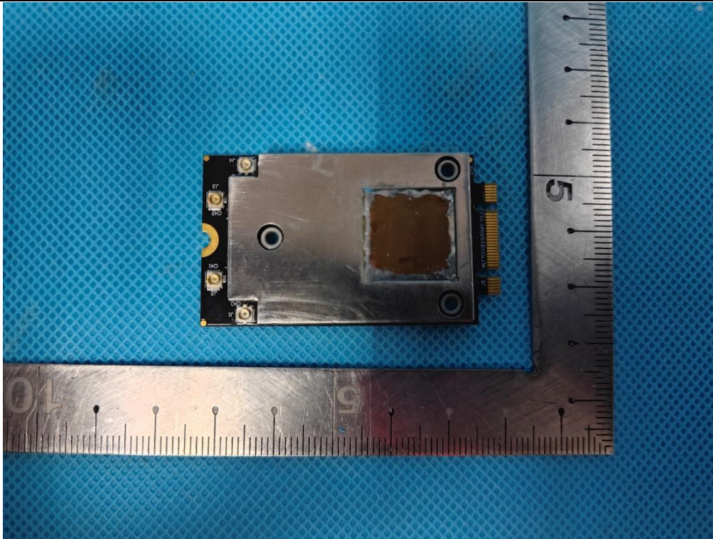
EUT Photo(2) - WLTB7000E5
