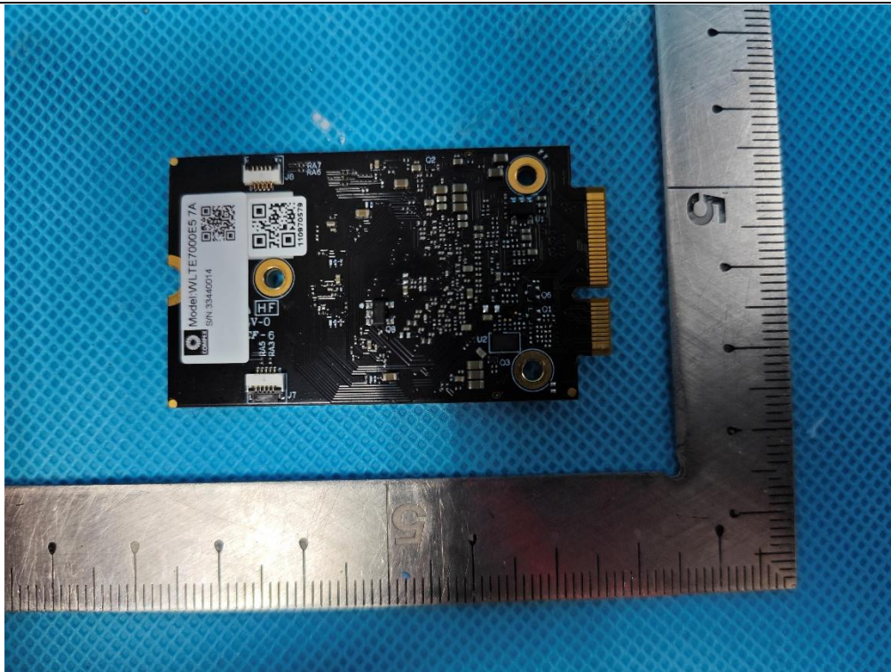
EUT Photo(12) - WLTE7000E5
