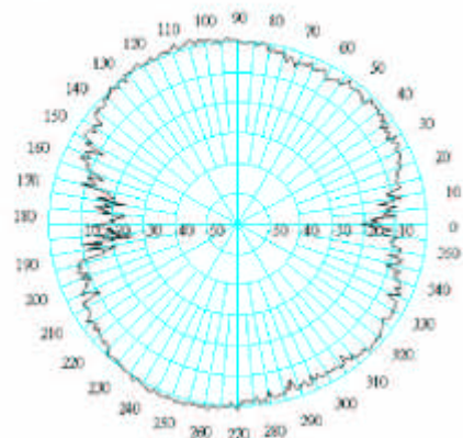
5.15~E-PLANE
