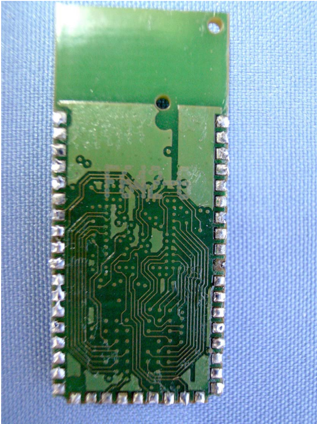
(9) EUT Photo
