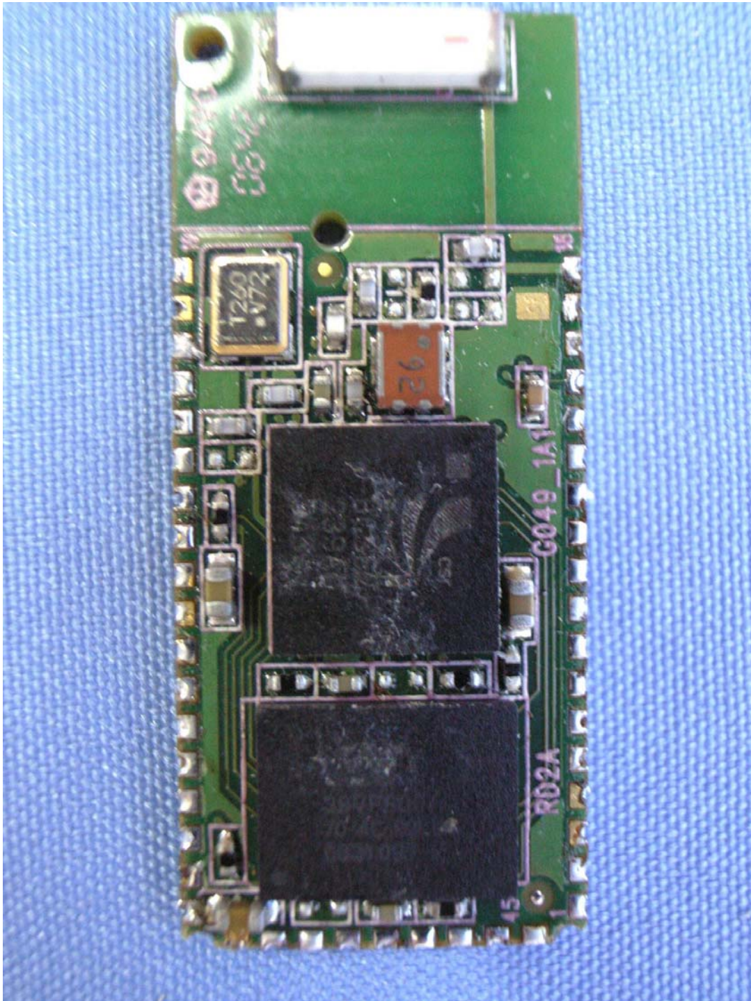
(8) EUT Photo
