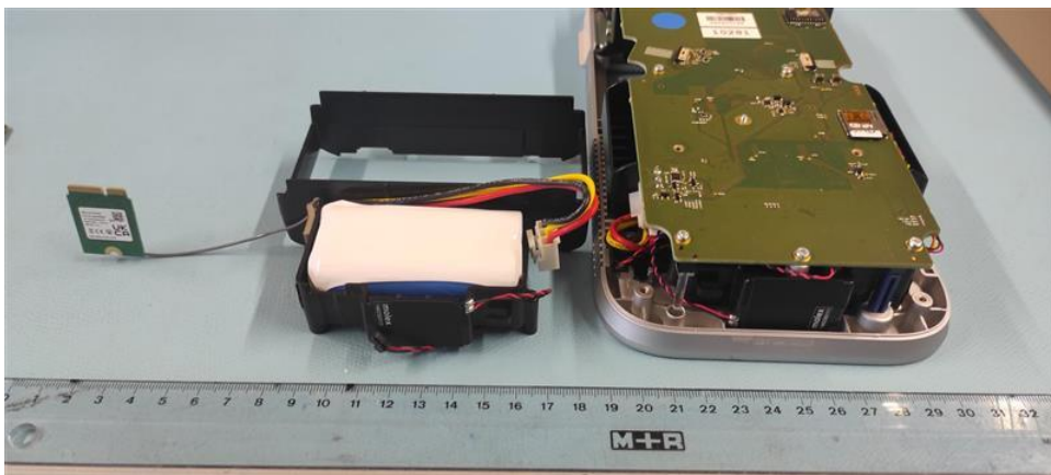
Wifi antenna & NFC antenna
