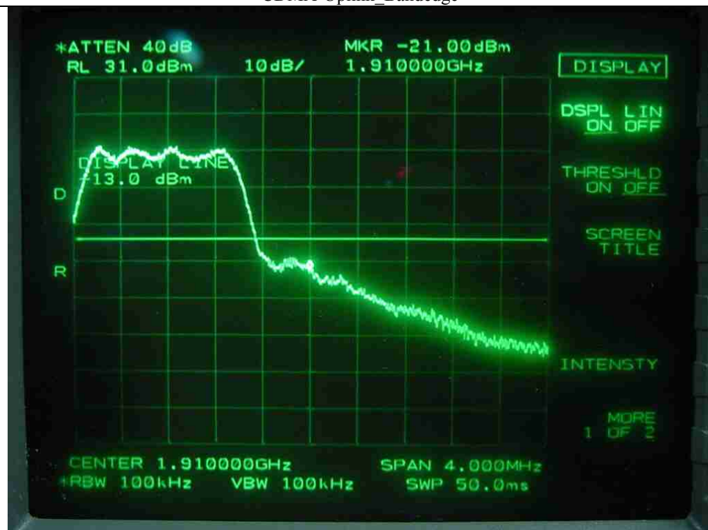
CDMA -Uplink_Bandedge
