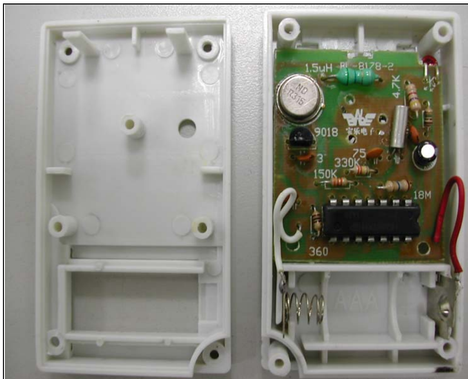
EUT Photo
