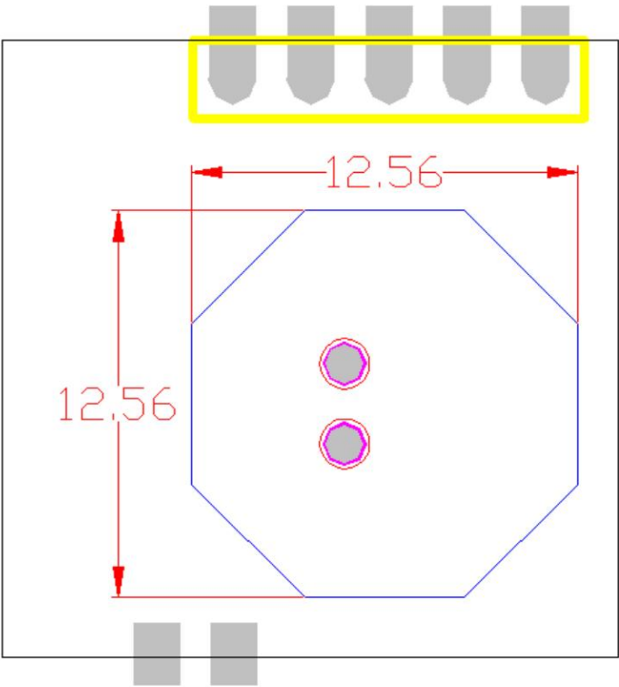
背视图
