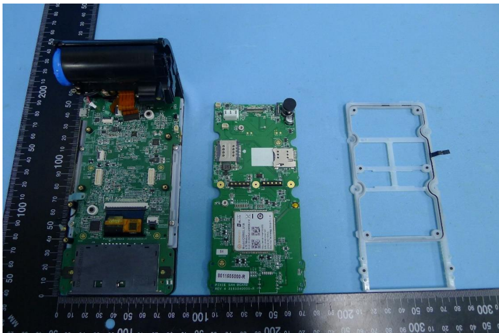
(6) EUT Photos
