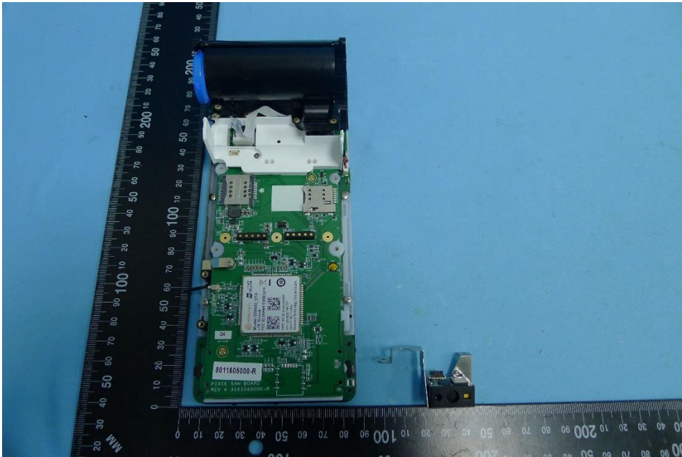
(3) EUT Photos
