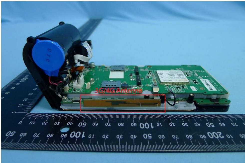
(5) EUT Photos
