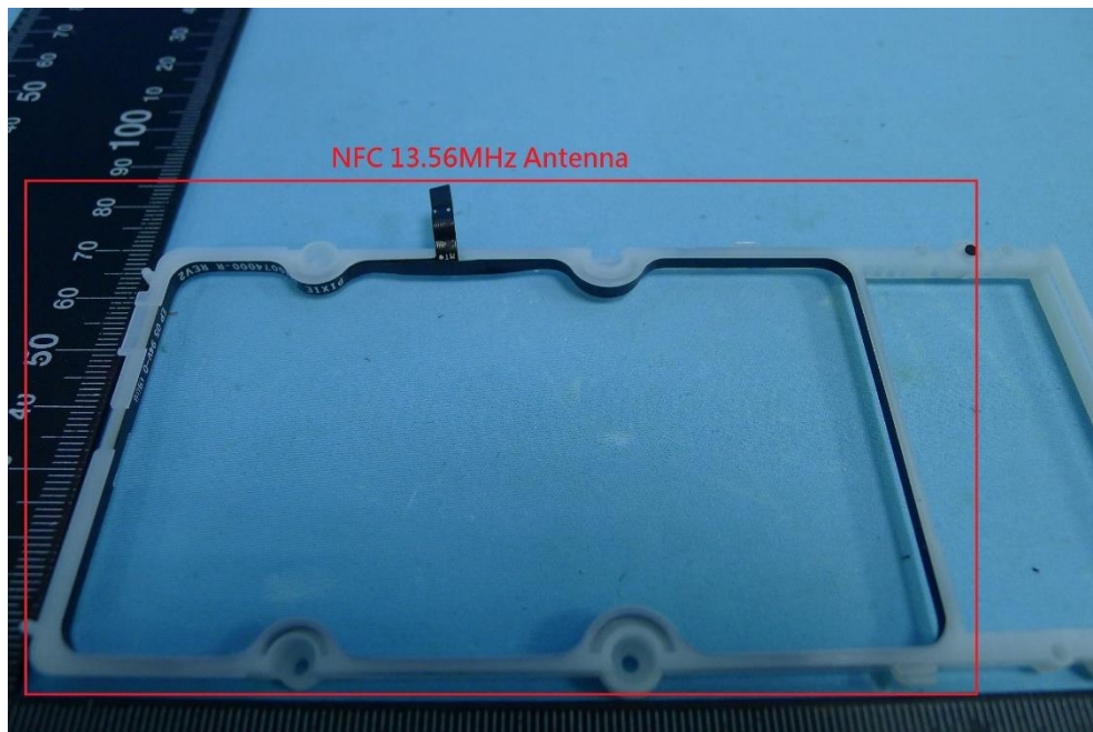
(13) EUT Photos
