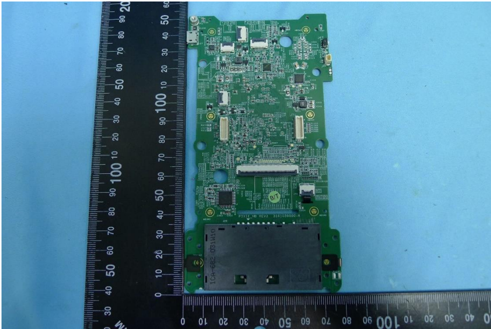
(15) EUT Photos
