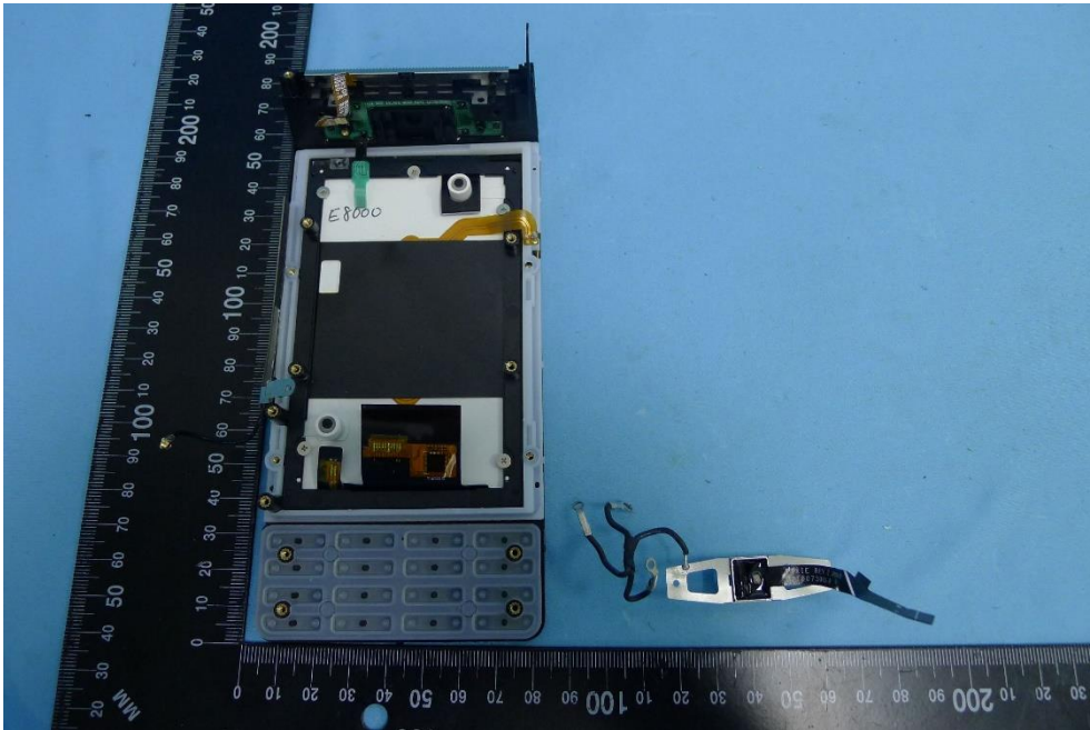
(21) EUT Photos
