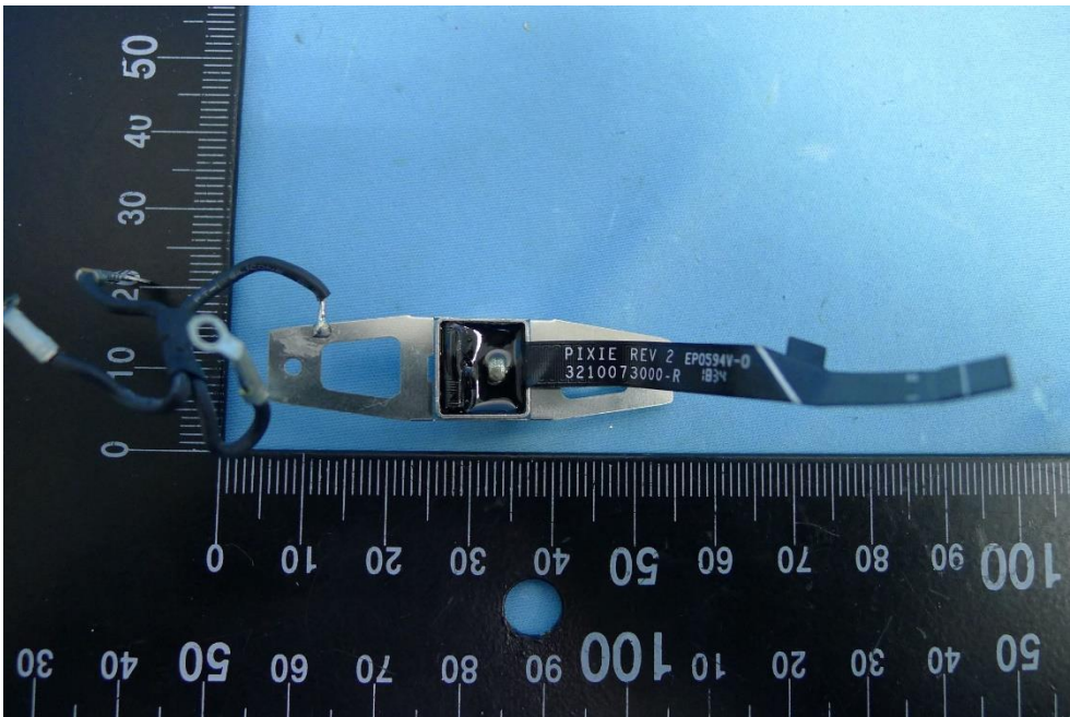
(22) EUT Photos
