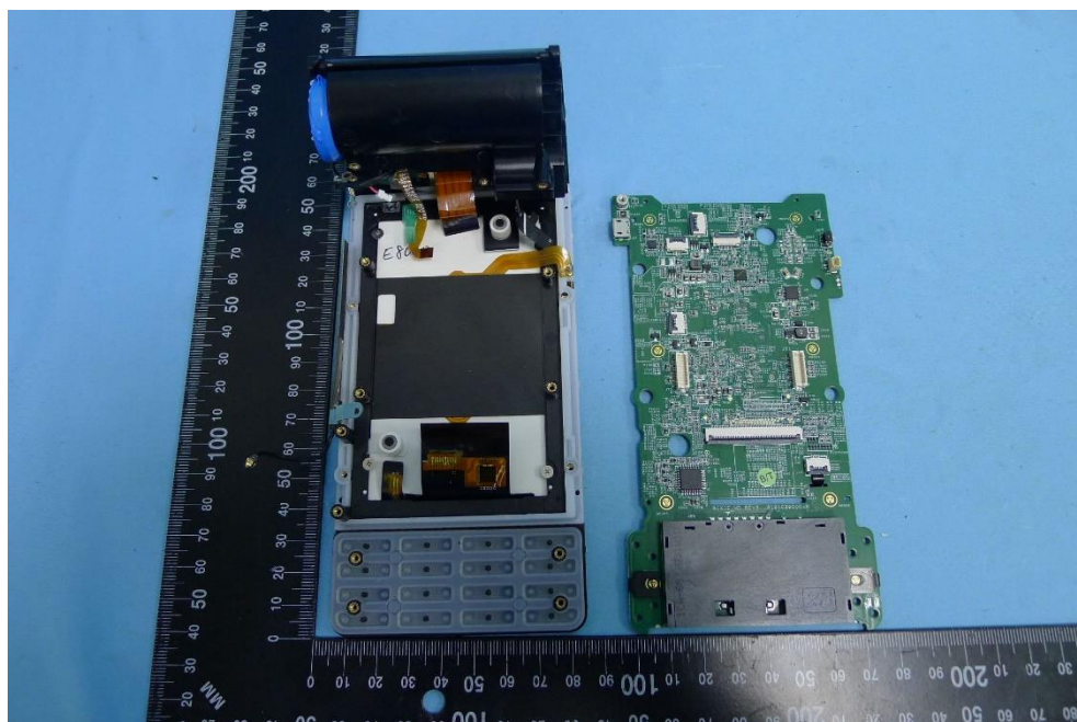
(14) EUT Photos
