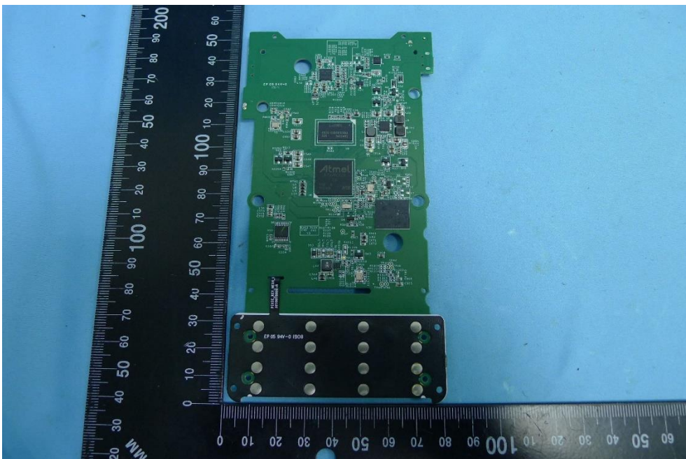
(16) EUT Photos
