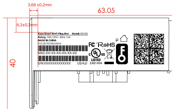
尺寸图
