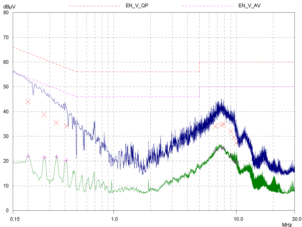
Neutral – PE
