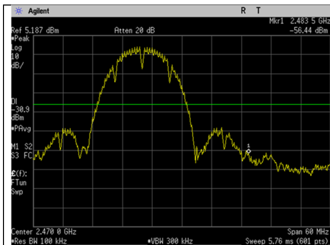
WIFI_High Ch_2462MHz_20MHz BW_b-mode_-20dBc_Upper Band Edge
