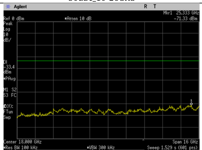
WIFI_Low Ch_2412MHz_20MHz BW_b-mode_-30dBc_10-26GHz
