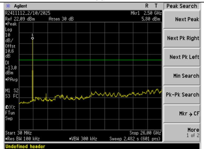
BLE_High Ch_2480MHz_2MBit_-20dBc_30MHz-26GHz
