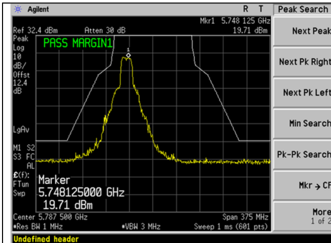
U-NII-3_5745MHz_20MHz BW_a-mode_Mask
