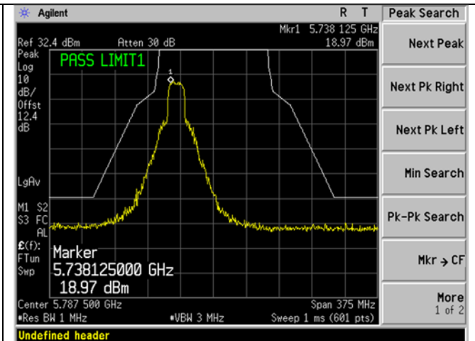
U-NII-3_5745MHz_20MHz BW_n-mode_Mask
