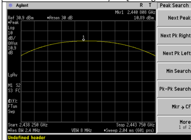
OUTPUT POWER \pi/4 -DQPSK mid
