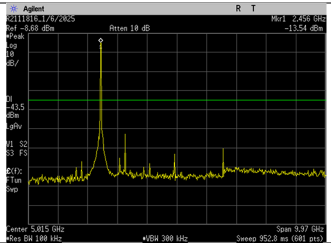
WIFI_High Ch_2462MHz_20MHz BW_n-mode_-30dBc_30MHz-10GHz
