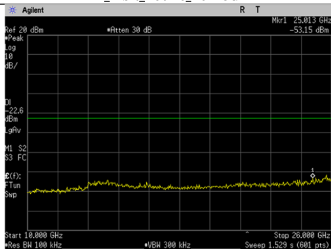
BLE_Mid CH_2440MHz_1MHz BW_Mbit_20dBc_10- 26GHz
