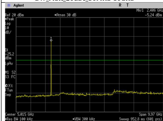
BLE_Low CH_2402MHz_2MHz BW_Mbit_20dBc_30MHz-10GHz
