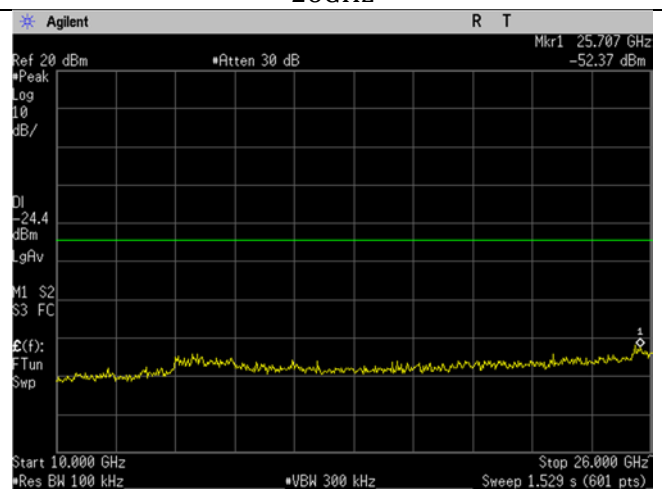
BLE_Mid CH_2440MHz_2MHz BW_Mbit_20dBc_10- 26GHz
