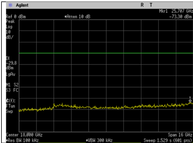
WIFI_High Ch_2462MHz_20MHz BW_b-mode_- 30dBc_10-26GHz
