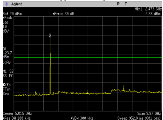
BLE_High CH_2480MHz_1MHz BW_Mbit_20dBc_30MHz-10GHz
