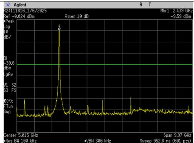
WIFI_Mid Ch_2437MHz_40MHz BW_n-mode_- 30dBc_30MHz-10GHz
