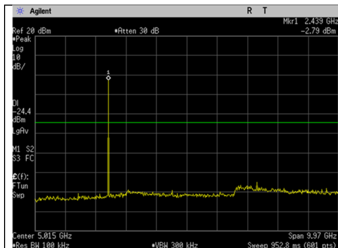
BLE_Mid CH_2440MHz_2MHz BW_Mbit_20dBc_30MHz-10GHz
