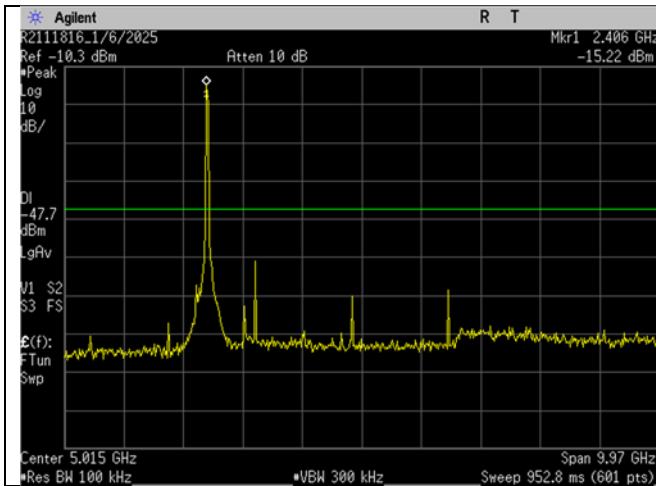
WIFI_Low Ch_2422MHz_40MHz BW_n-mode_- 30dBc_30MHz-10GHz
