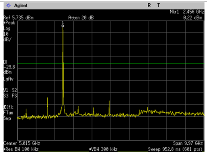
WIFI_High Ch_2462MHz_20MHz BW_b-mode_- 30dBc_30MHz-10GHz
