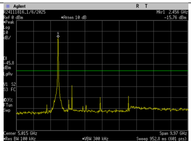
WIFI_High Ch_2452MHz_40MHz BW_n-mode_-30dBc_30MHz-10GHz
