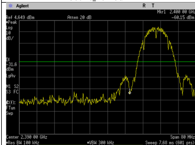
WIFI_Low Ch_2412MHz_20MHz BW_b-mode_-30dBc_Lower Band Edge
