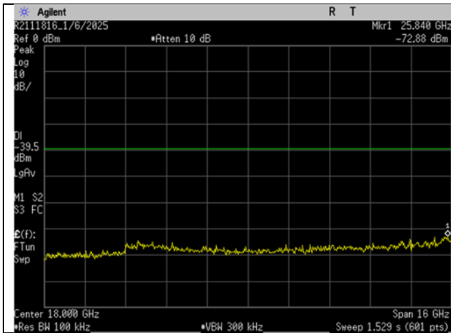
WIFI_Mid Ch_2437MHz_20MHz BW_n-mode_- 30dBc_10-26GHz
