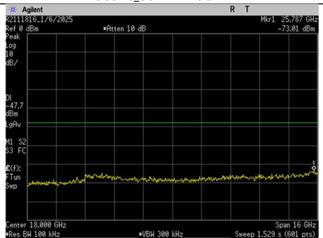
WIFI_Low Ch_2422MHz_40MHz BW_n-mode_- 30dBc_10-26GHz
