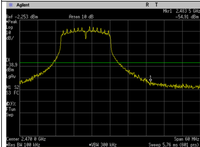
WIFI_High Ch_2462MHz_20MHz BW_g-mode_- 20dBc_Upper Band Edge
