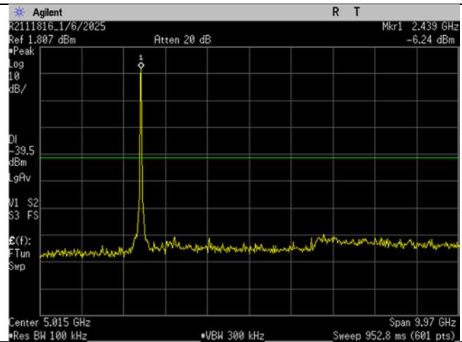
WIFI_Mid Ch_2437MHz_20MHz BW_n-mode_- 30dBc_30MHz-10GHz
