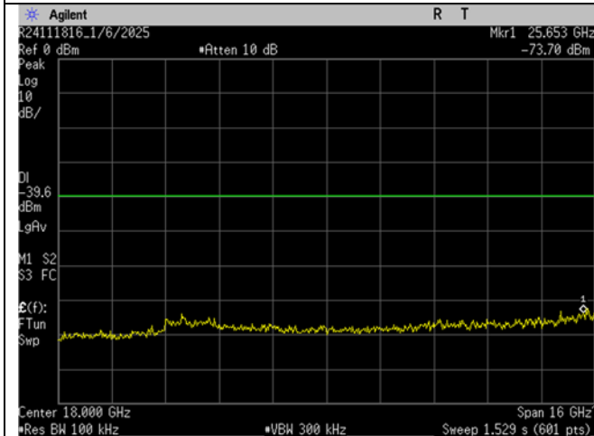
WIFI_Mid Ch_2437MHz_40MHz BW_n-mode_- 30dBc_10-26GHz
