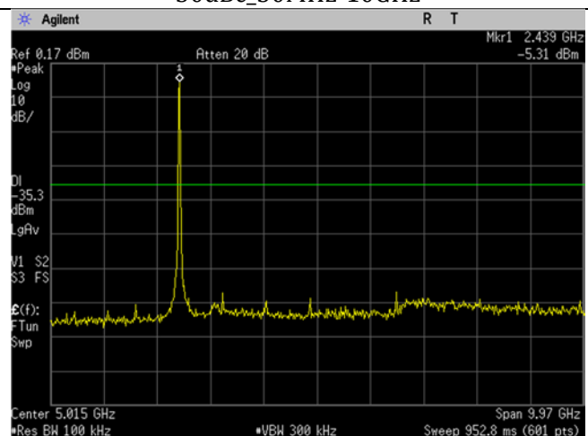
WIFI_Mid Ch_2437MHz_20MHz BW_g-mode_- 30dBc_30MHz-10GHz
