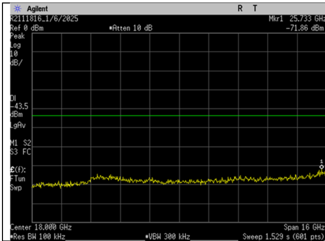
WIFI_High Ch_2462MHz_20MHz BW_n-mode_-30dBc_10-26GHz
