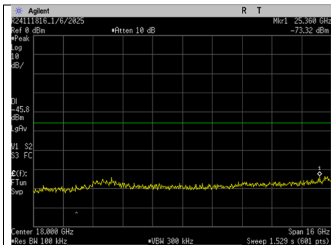
WIFI_High Ch_2452MHz_40MHz BW_n-mode_-30dBc_10-26GHz
