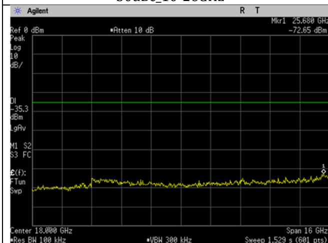
WIFI_Mid Ch_2437MHz_20MHz BW_g-mode_- 30dBc_10-26GHz
