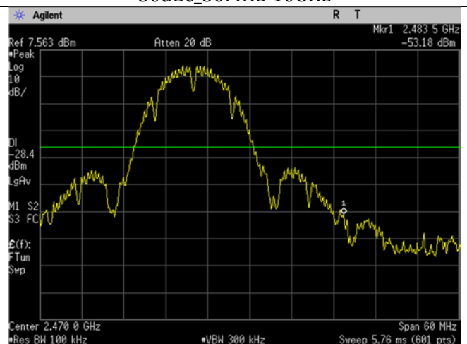
WIFI_High Ch_2462MHz_20MHz BW_b-mode_-30dBc_Upper Band Edge
