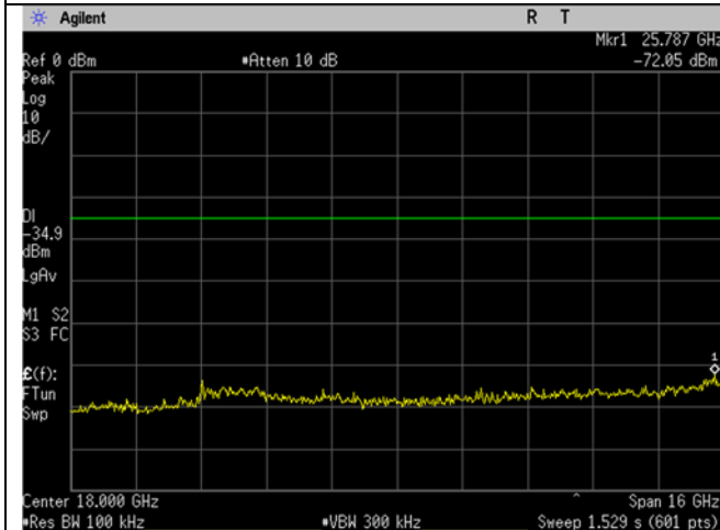
WIFI_Low Ch_2412MHz_20MHz BW_b-mode_-30dBc_10-26GHz
