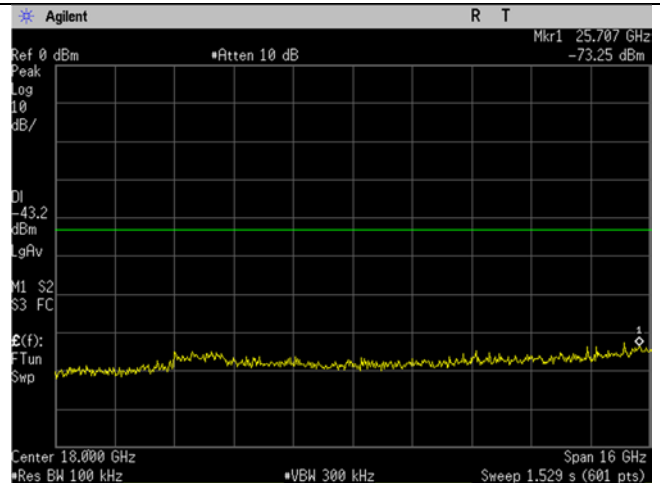
WIFI_High Ch_2462MHz_20MHz BW_g-mode_- 30dBc_10-26GHz
