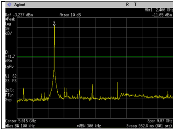
WIFI_Low Ch_2412MHz_20MHz BW_g-mode_- 30dBc_30MHz-10GHz
