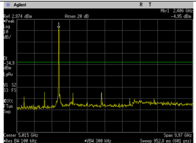
WIFI_Low Ch_2412MHz_20MHz BW_b-mode_-30dBc_30MHz-10GHz
