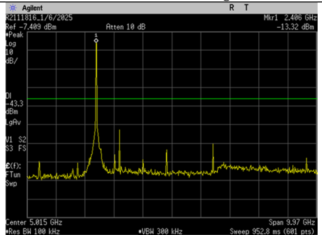
WIFI_Low Ch_2412MHz_20MHz BW_n-mode_- 30dBc_30MHz-10GHz
