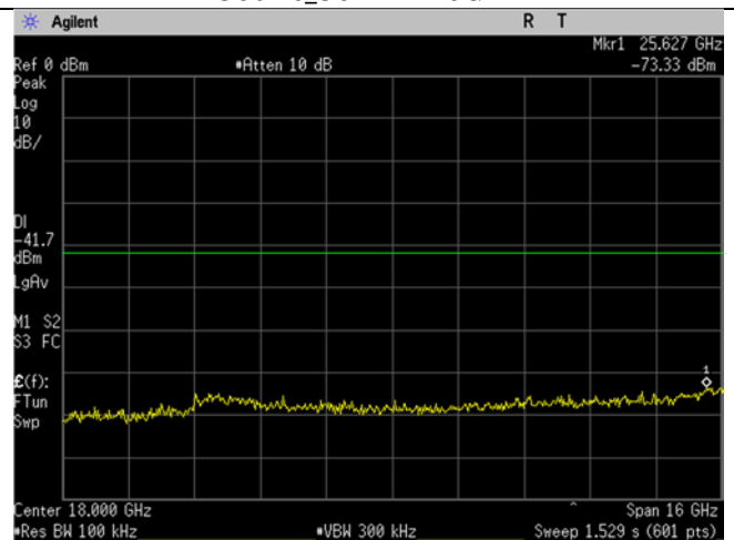
WIFI_Low Ch_2412MHz_20MHz BW_g-mode_-30dBc_10-26GHz
