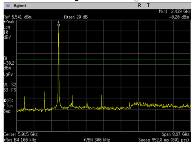
WIFI_Mid Ch_2437MHz_20MHz BW_b-mode_- 30dBc_30MHz-10GHz
