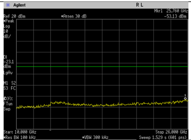
BLE_High CH_2480MHz_2MHz BW_Mbit_20dBc_10-26GHz
