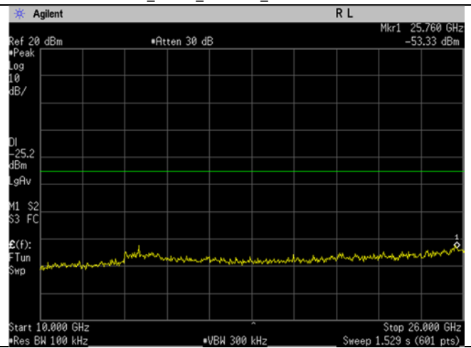
BLE_Low CH_2402MHz_2MHz BW_Mbit_20dBc_10- 26GHz
