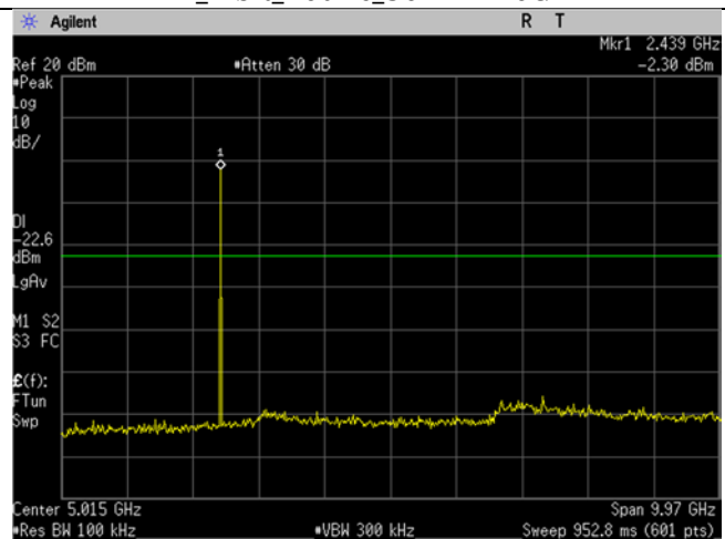
BLE_Mid CH_2440MHz_1MHz BW_Mbit_20dBc_30MHz-10GHz
