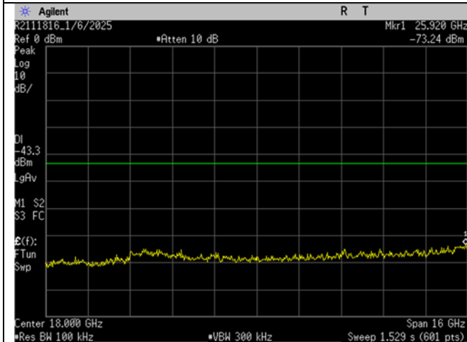
WIFI_Low Ch_2412MHz_20MHz BW_n-mode_- 30dBc_10-26GHz
