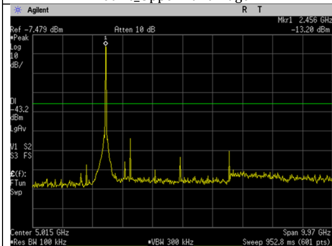
WIFI_High Ch_2462MHz_20MHz BW_g-mode_- 30dBc_30MHz-10GHz
