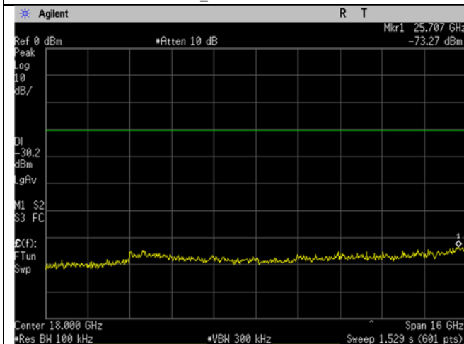
WIFI_Mid Ch_2437MHz_20MHz BW_b-mode_- 30dBc_10-26GHz
