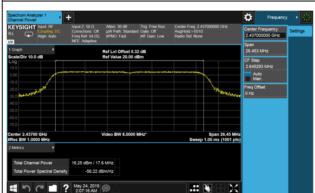
802.11n-HT20 2437MHz
