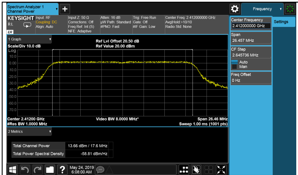
802.11n-HT20 2412MHz
