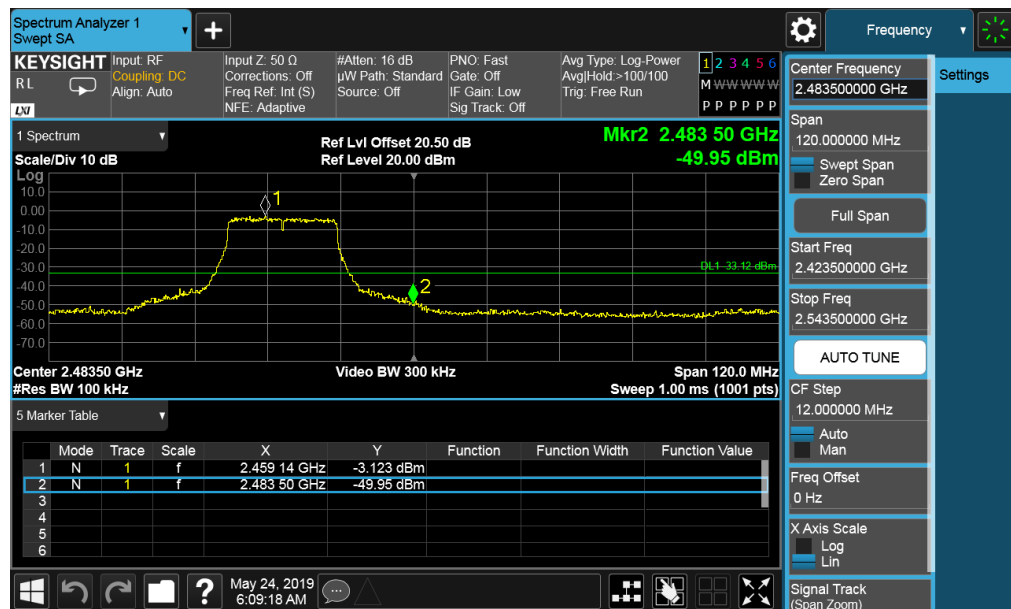
802.11n-HT20-2462MHz
