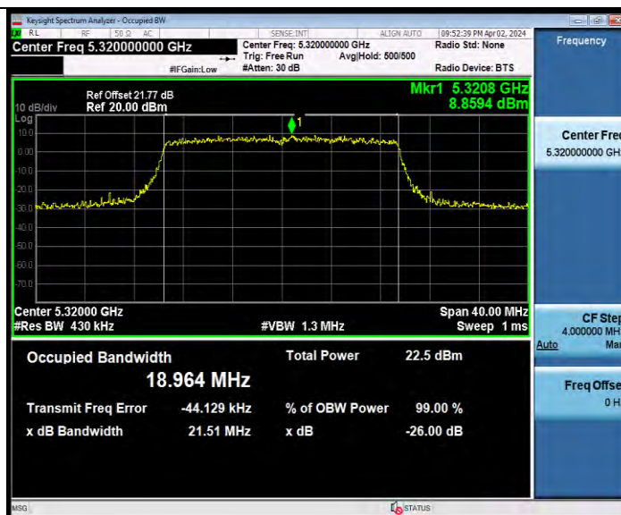
11AX20MIMO_Ant6_5320
