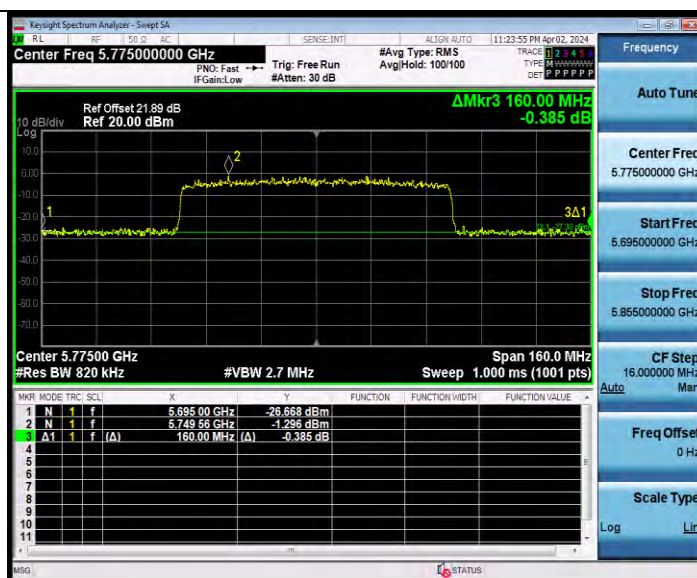
11AX80MIMO_Ant6_5775
