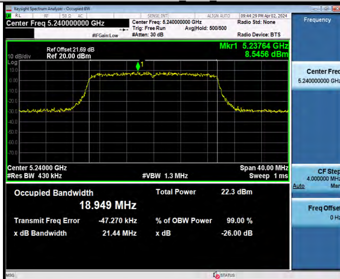
11AX20MIMO_Ant5_5260
