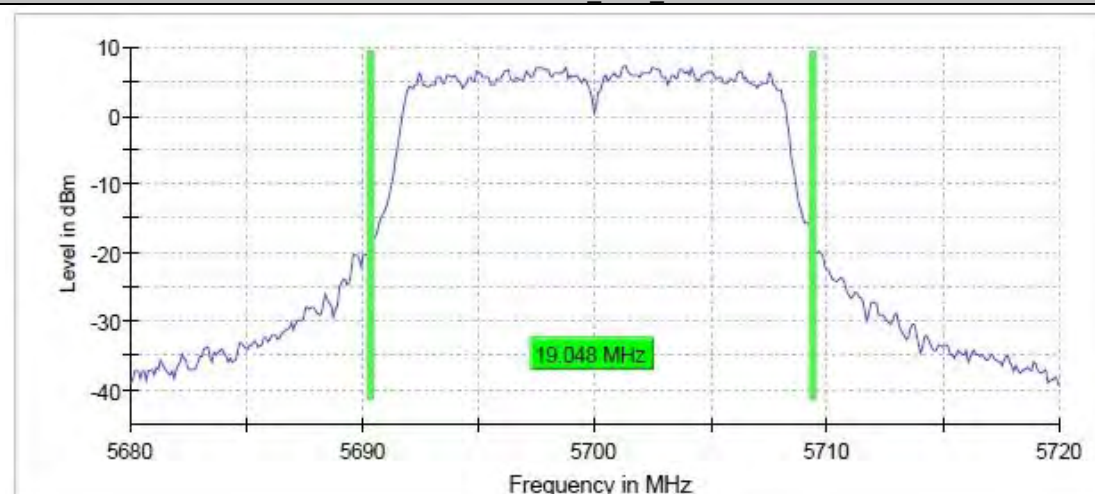
11A_Ant6_5700
