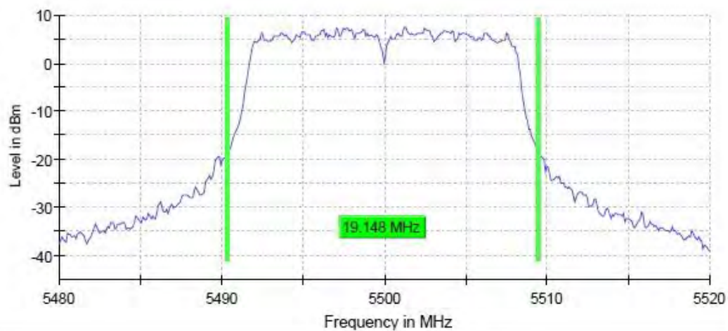
11A_Ant6_5500
