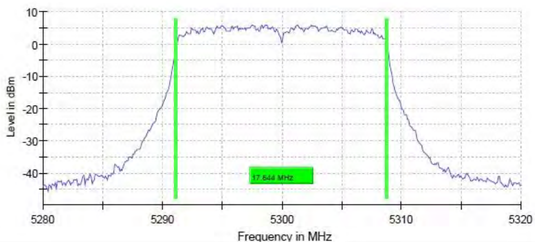
11AC20 Ant6 5300
