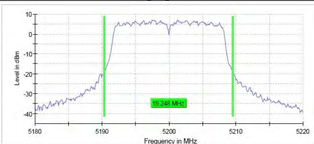
11A_Ant6_5200
