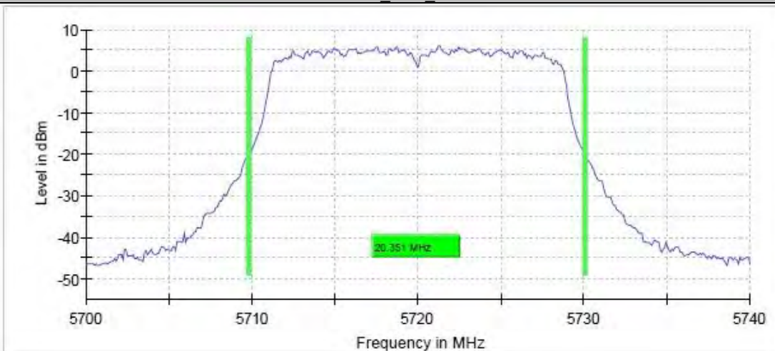
11AC20_Ant6_5720
