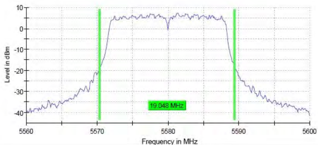
11A_Ant6_5580
