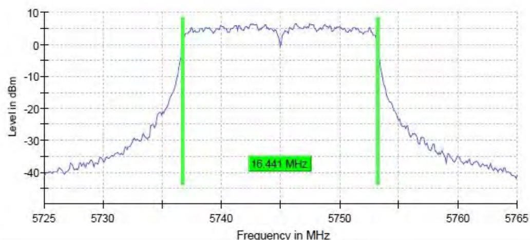
11A_Ant6_5745
