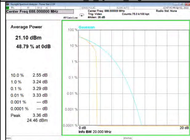
Band 71_1_Q16_High
