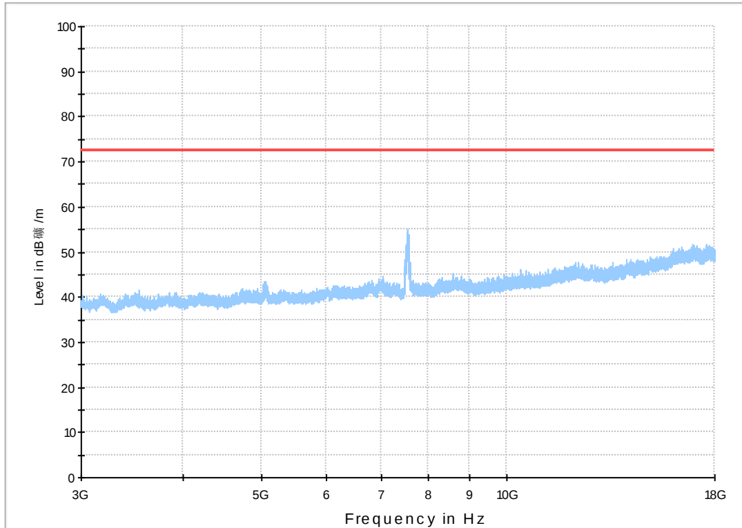
R SE_Erisson_3-18G_FCC
