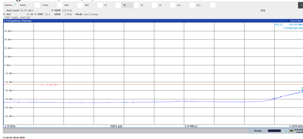
Diagram 2.11b, TM6, B, Port A:
