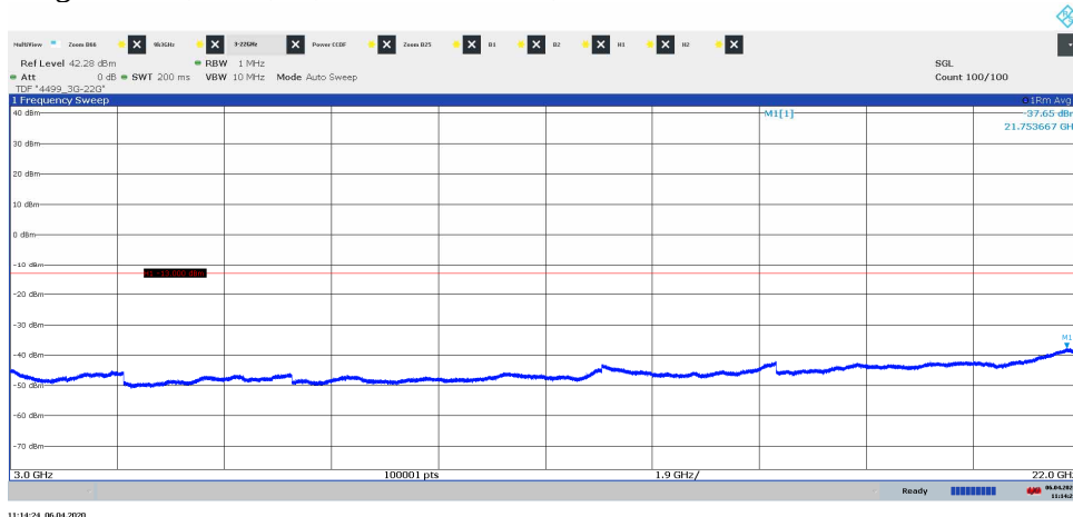
Diagram 3.2b, TM1, M, 3 GHz – 22 GHz, Port A:
