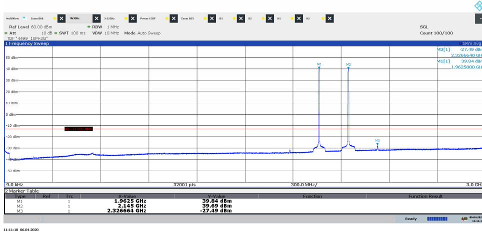
Diagram 3.2a, TM1, M, 9 kHz – 3 GHz, Port A:
