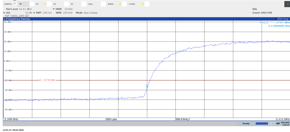
Diagram 2.22a, TM1, B, Port D:
