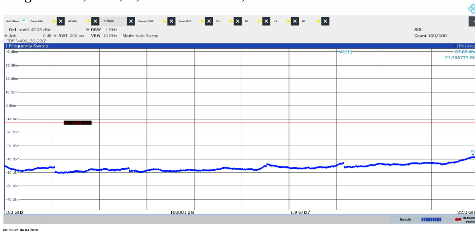
Diagram 3.1b, TM1, B, 3 GHz – 22 GHz, Port A:
