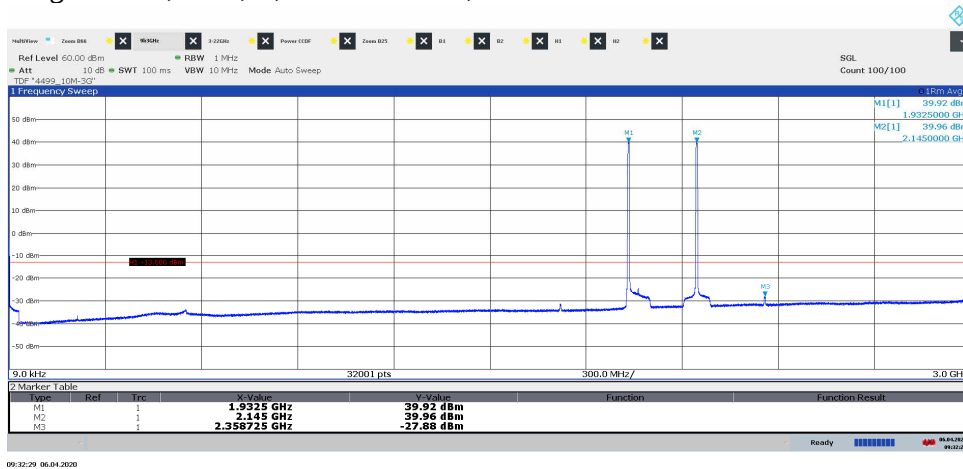
Diagram 3.1a, TM1, B, 9 kHz – 3 GHz, Port A:
