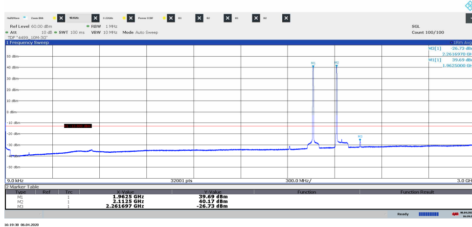
Diagram 3.10a, TM1, B, 9 kHz – 3 GHz, Port A:
