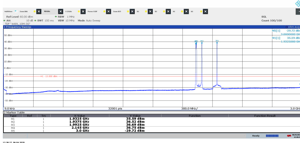
Diagram 3.7a, TM1, Bim, 9 kHz – 3 GHz, Port A:
