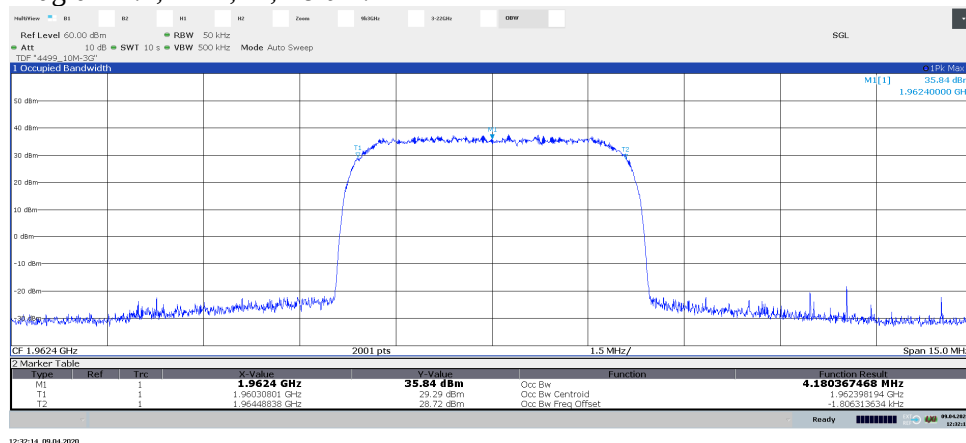
Diagram 1.2, TM1, M, Port A:
