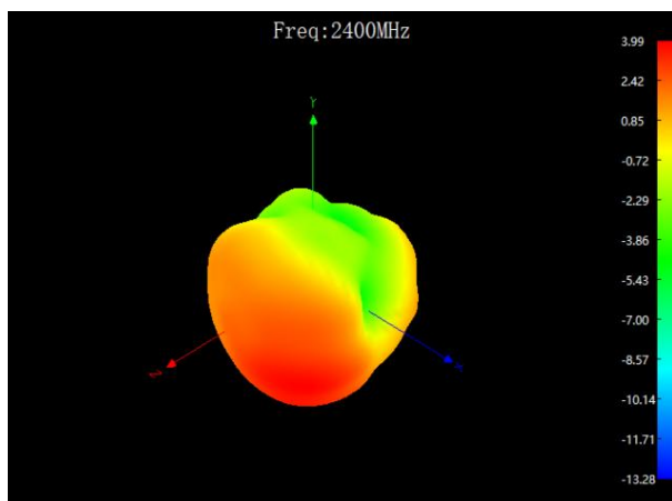
天线 2400MHz 3D-Horizontal Pattern
