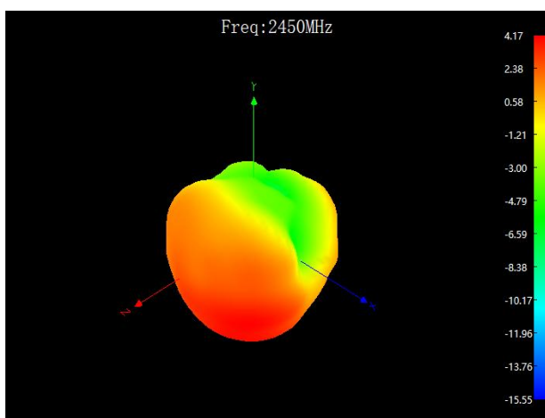
天线 2450MHz 3D-Vertical Pattern
