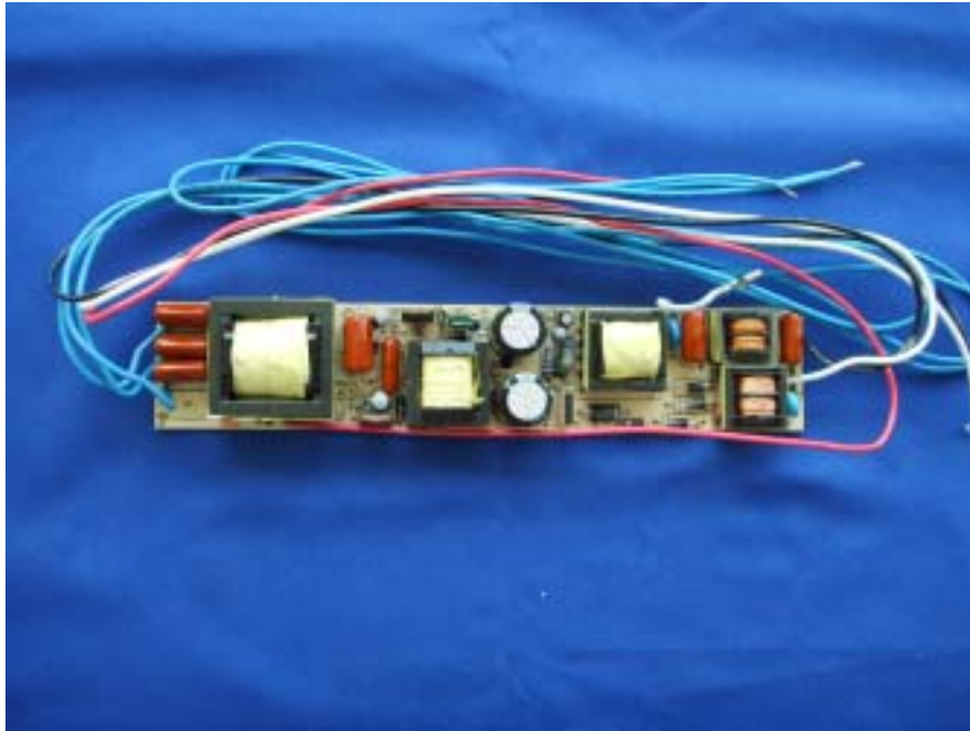
EBT08-332H-MS1-00 –Components View
