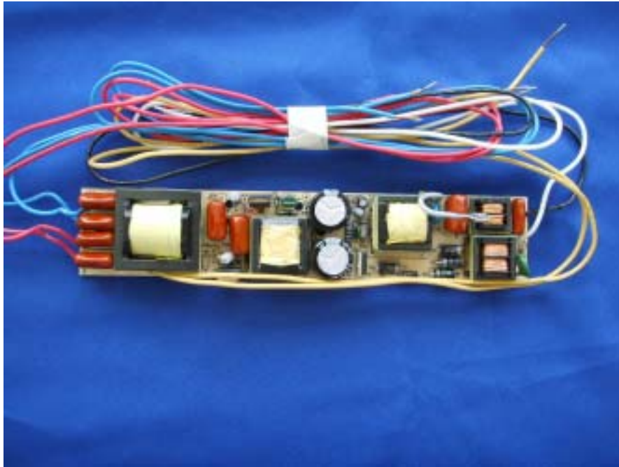
EBT08-432H-MS1-00 –Components View
