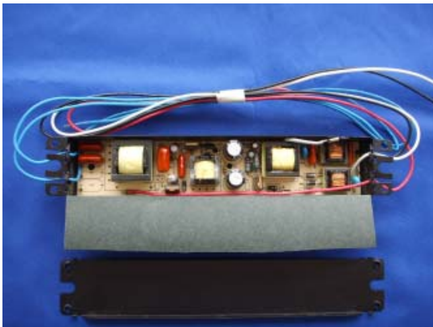
EBT08-232H-MS1-00 –Uncovered View
