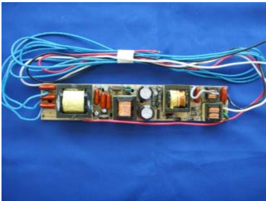
EBT08-332UH-MS1-00 –Components View
