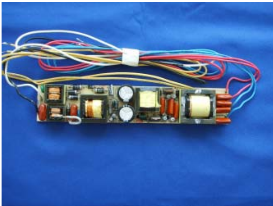
EBT08-432UH-MS1-00 –Components View
