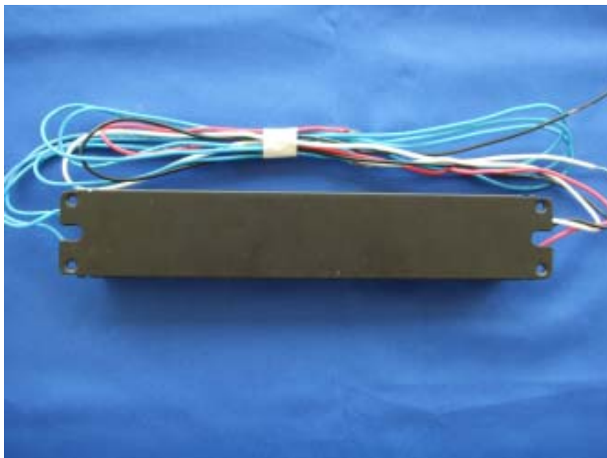
EBT08-332UH-MS1-00 – Back View
