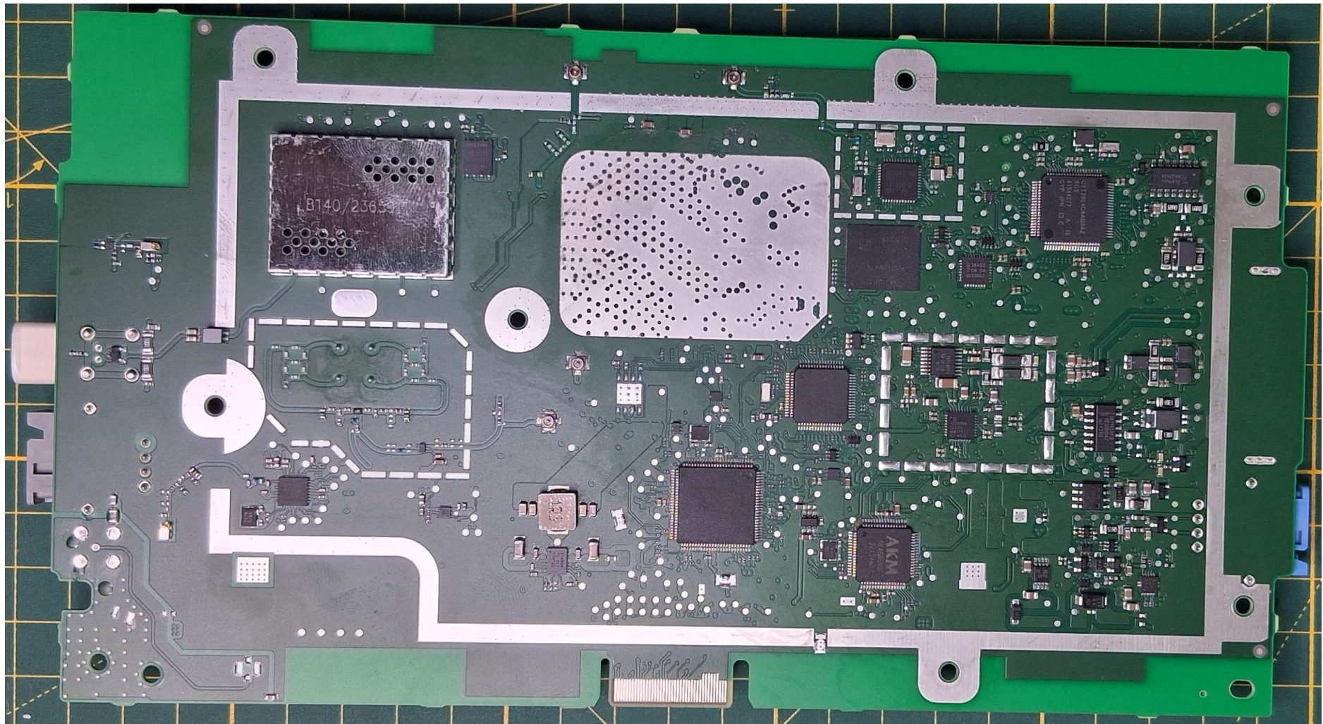
Bottom side
