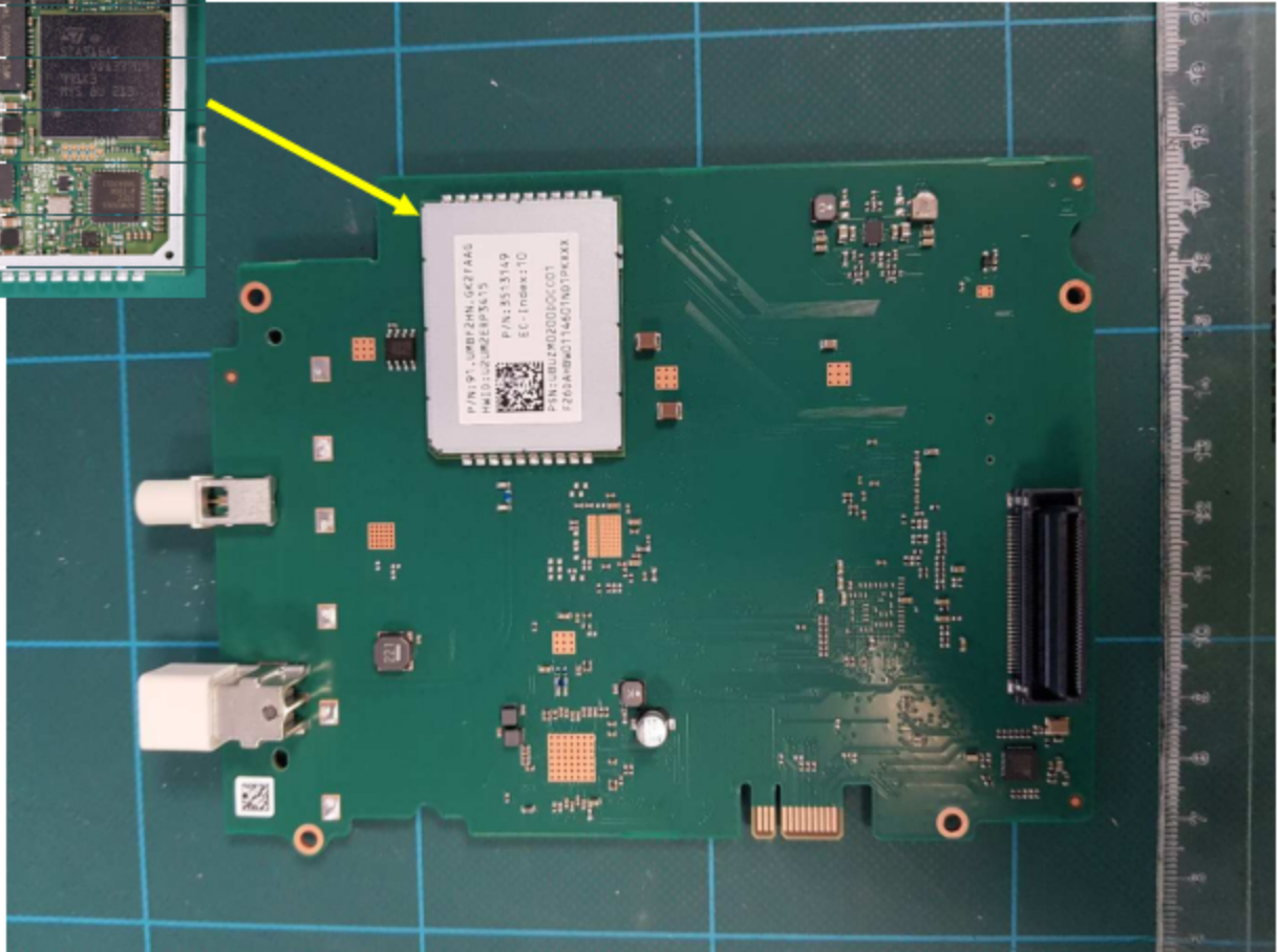
PCBA 4065 TUNER CSB D2 C M239
