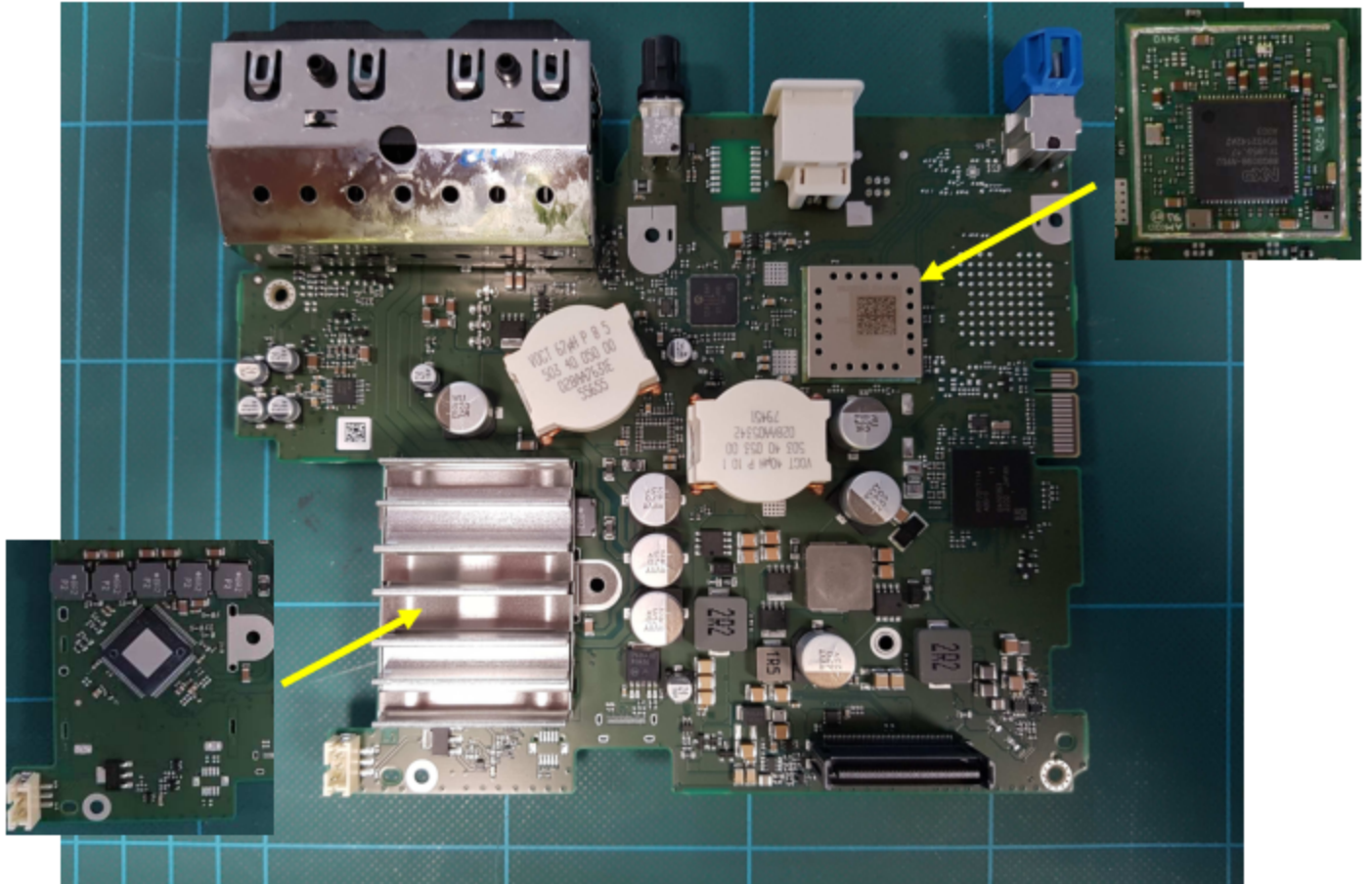
PCBA 4010 MAIN BB D11 M649
