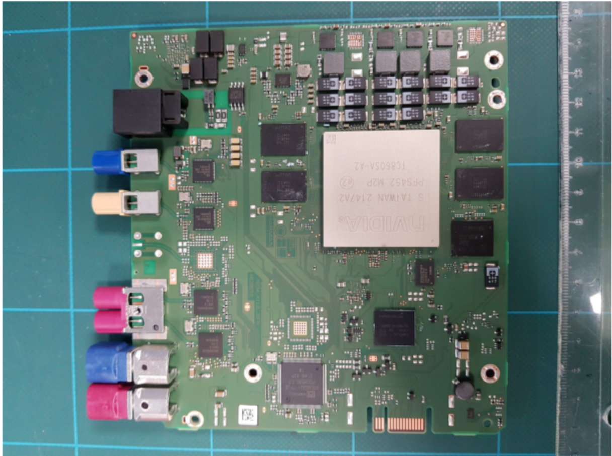
PCBA 4110 MAIN MMB 3TPC D11 M654
