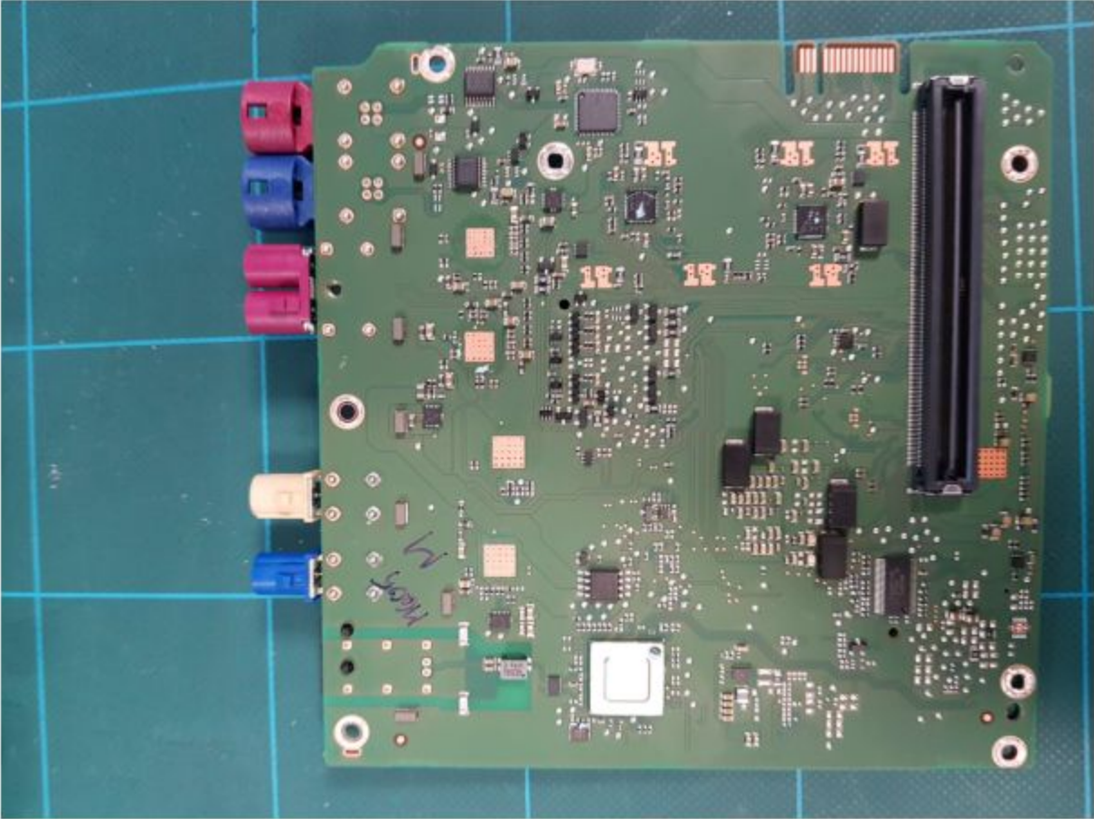
PCBA 4110 MAIN MMB 16GB D11 M605
