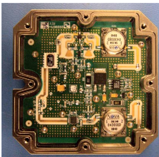
Fig 5 – EXVR 4300-05M1 RF UNIT
