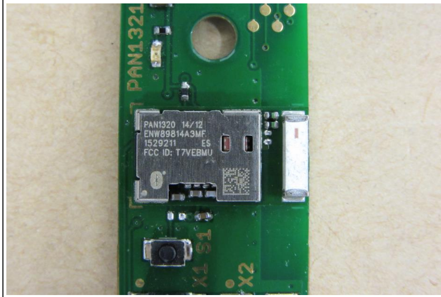
EUT Modul Label
