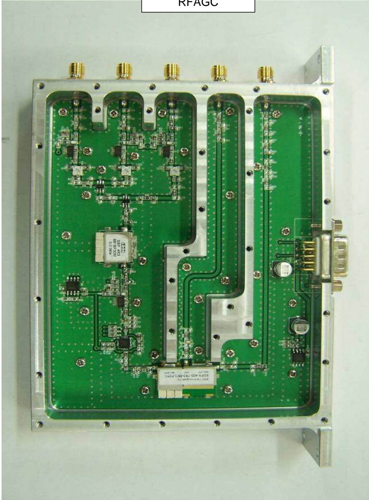
RFAGC
