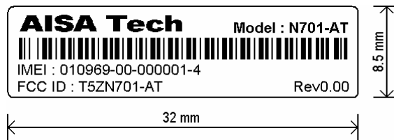
IMEI label on the N701-AT PCB bottom
