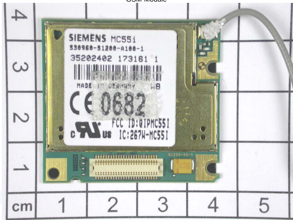
GSM-Module
