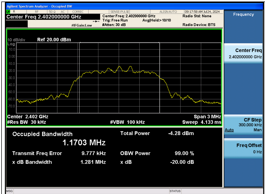
Test_Graph_EDR_ANT1_2402_2Mbps_OBW
