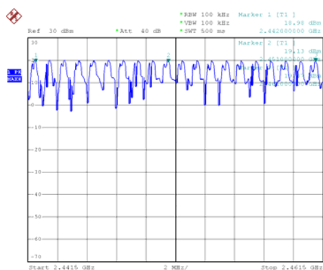
2442-2461MHz
