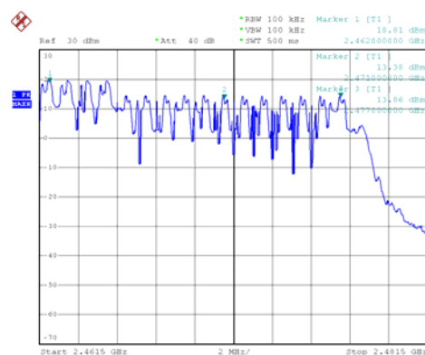
2462-2477MHz
