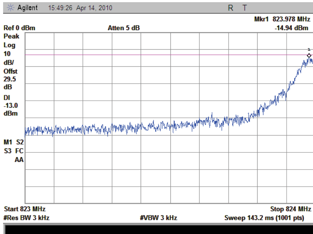
(Plot A: GSM Channel = 128)
