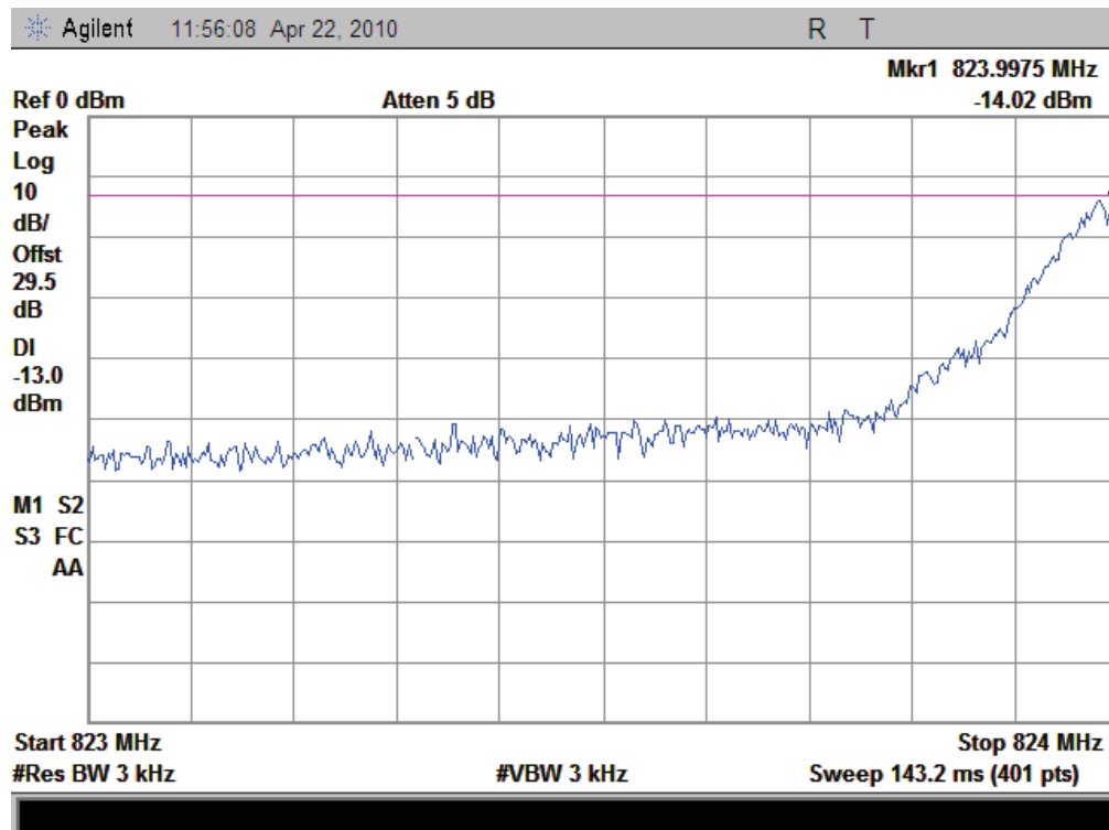
(Plot A: GPRS Channel = 128)
