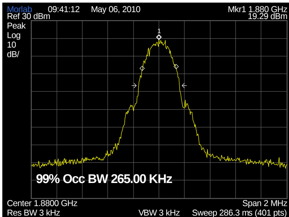
(Plot B: GSM 1900MHz Channel = 661)
