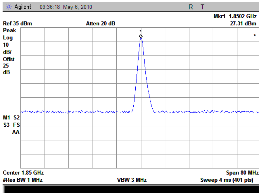
(Plot A: GSM 1900MHz Channel = 512)
