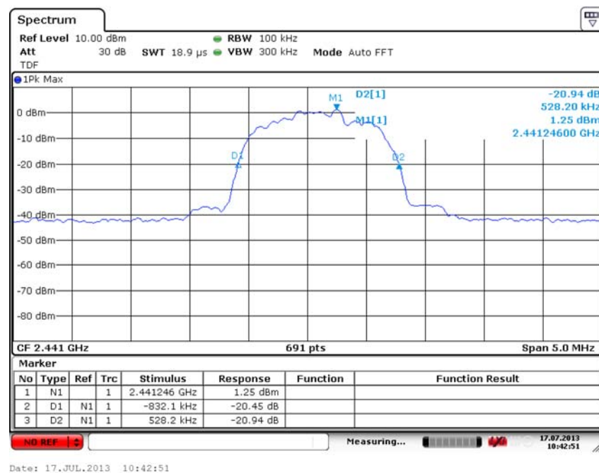
Fig. 70 Occupied 20dB Bandwidth ( \pi/4 DQPSK, Ch 39)
