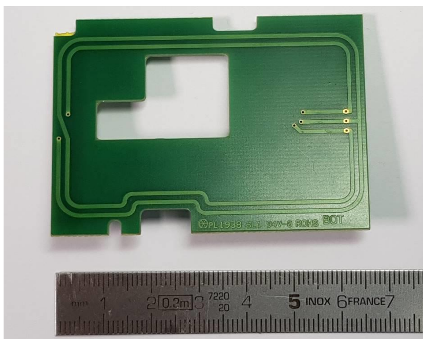
IMS antenna Bot (CAR_1000006460)
