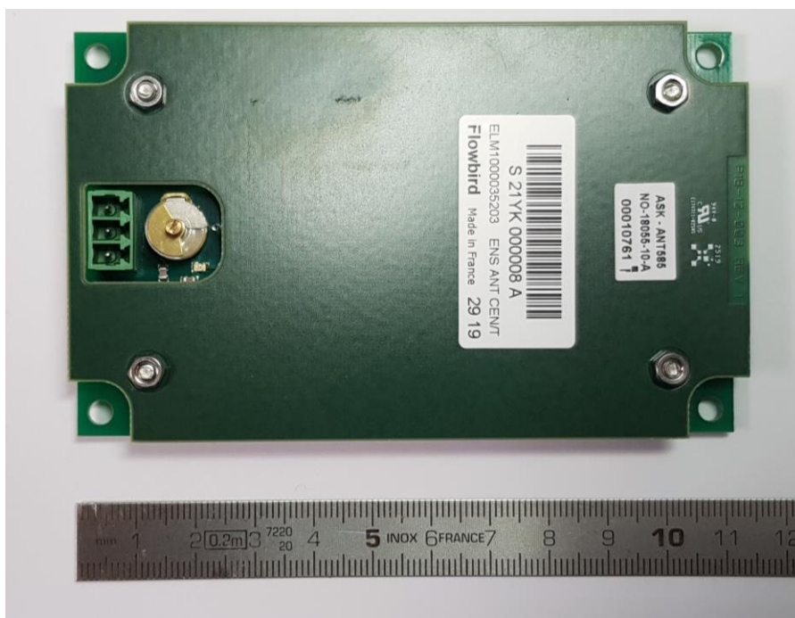
Paragon antenna Bot (ELM_1000035203)
