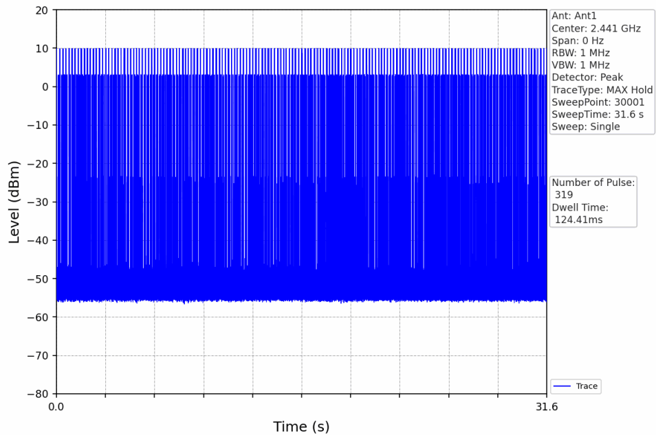
8DPSK_3DH1_HOPP_Ant1_NTNV
