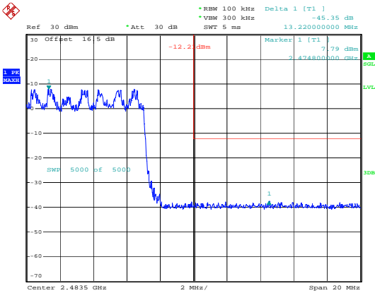
3EDR_DH1_Hopping_Upper
