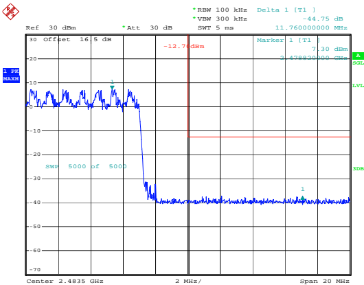
2EDR_DH1_Hopping_Upper
