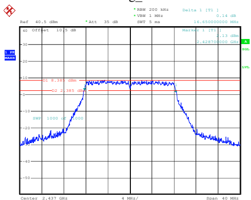
802.11g_2437MHz
