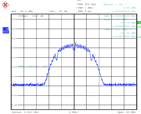
802.11b_2412MHz
