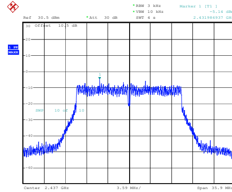
802.11n20_2437MHz
