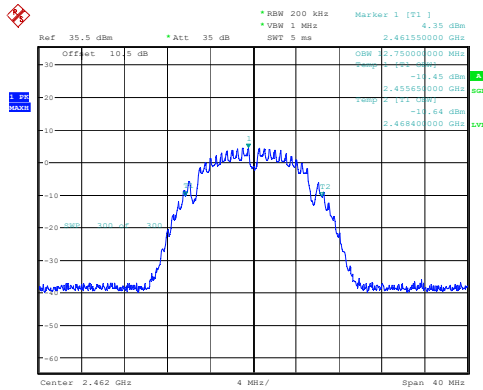
802.11b_2462MHz
