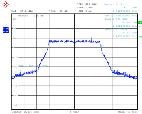
802.11g_2437MHz
