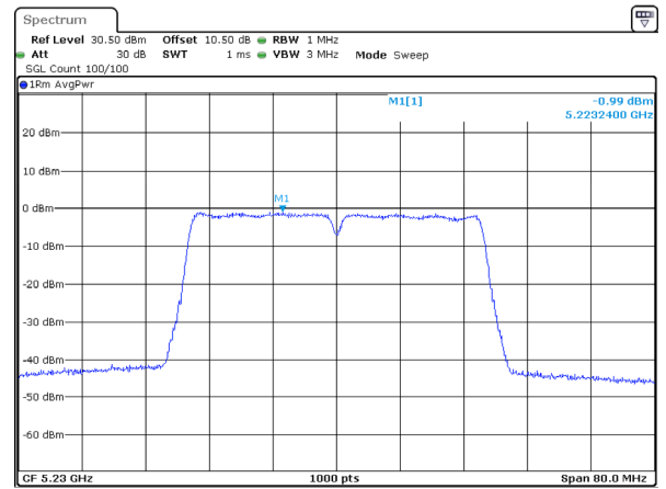
802.11ac40_5230MHz
