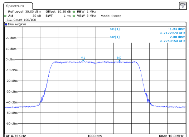
802.11ax20_5720MHz_RU_Full
