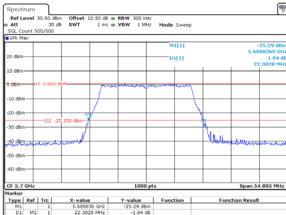
802.11ac20_5700MHz
