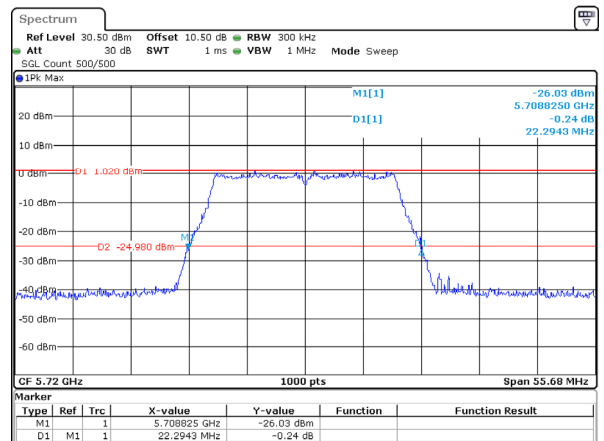
802.11ac20_5720MHz
