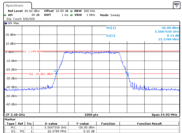
802.11ac20_5580MHz
