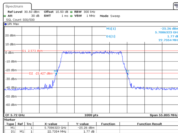
802.11ax20_5720MHz_RU_Full
