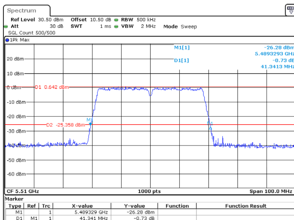
802.11ac40_5510MHz
