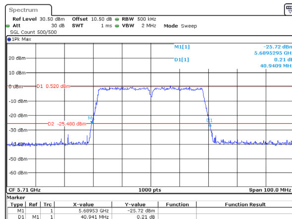
802.11ac40_5710MHz
