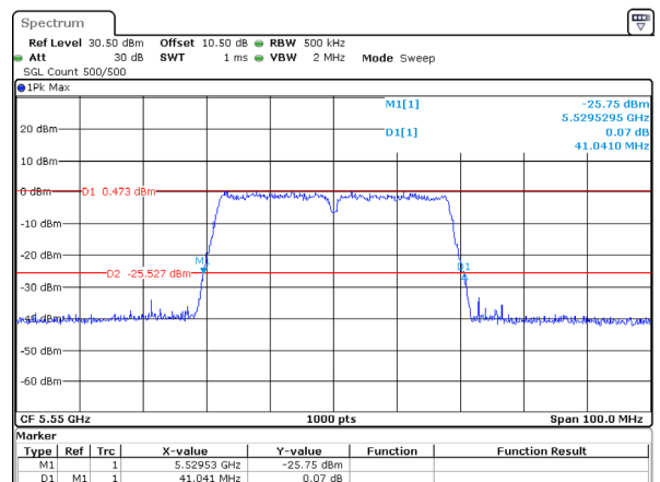
802.11ac40_5550MHz
