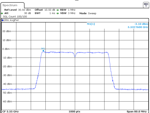
802.11ac40_5550MHz
