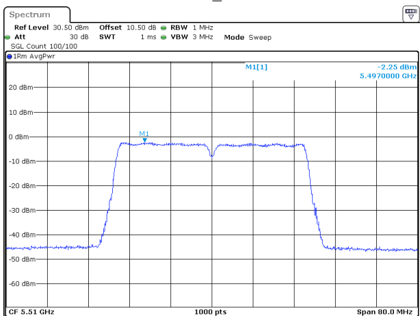
802.11ac40_5510MHz
