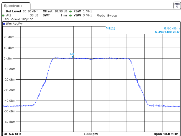
802.11ac20_5500MHz
