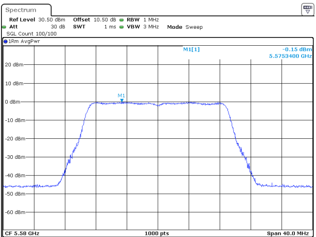
802.11ac20_5580MHz
