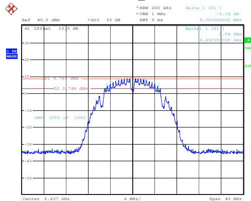
802.11b_2437MHz
