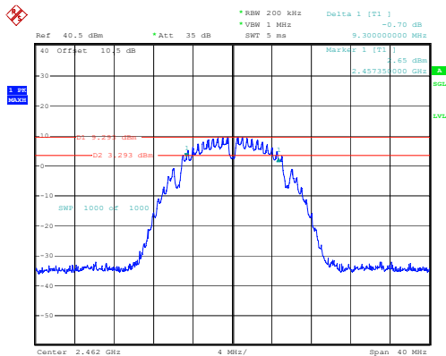
802.11b_2462MHz
