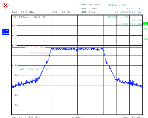
802.11g_2437MHz
