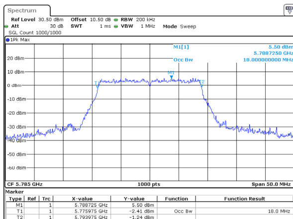
802.11ac20_5785MHz 18MHz
