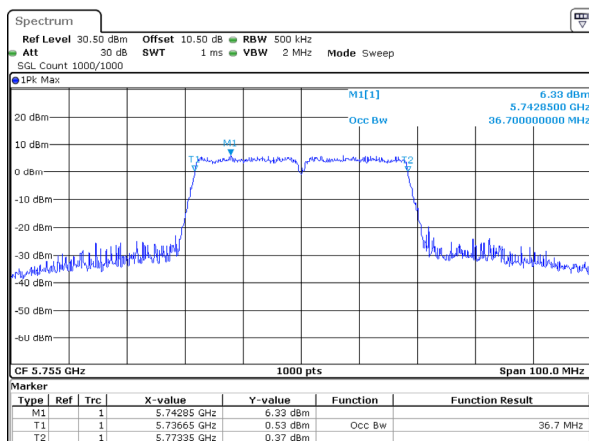
802.11ac40_5755MHz 36.700MHz
