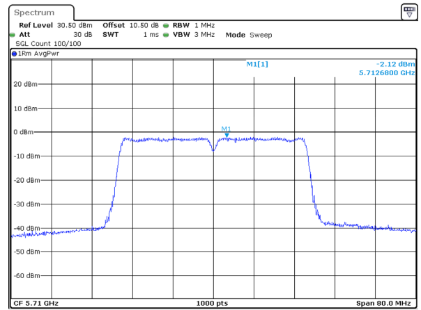
802.11ac40_5710MHz
