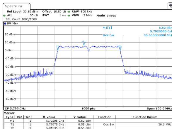
802.11ac40_5795MHz 36.600MHz
