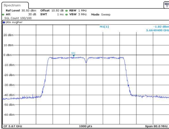
802.11ac40_5670MHz
