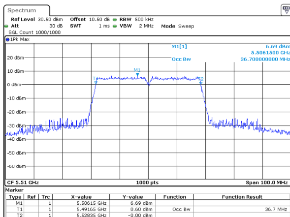
802.11ac40_5510MHz 36.700MHz
