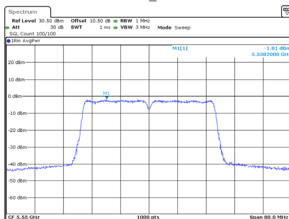
802.11ac40_5550MHz
