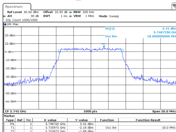
802.11ac20_5745MHz 18MHz
