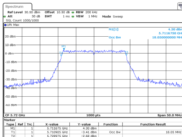
802.11ac20_5720MHz 18.050MHz
