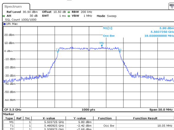
802.11ac20_5500MHz 18.050MHz
