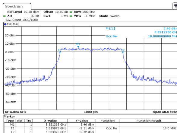
802.11ac20_5825MHz 18MHz
