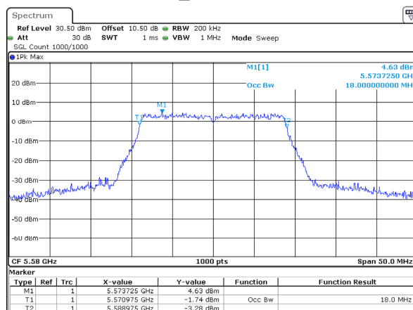
802.11ac20_5580MHz 18MHz
