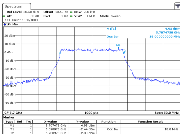
802.11ac20_5700MHz 18MHz
