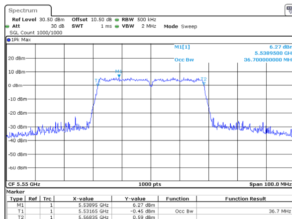
802.11ac40_5550MHz 36.700MHz
