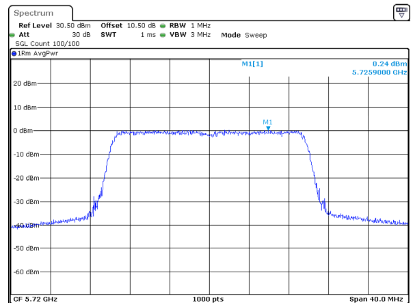
802.11ax20_5720MHz_RU_Full
