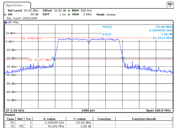
802.11ac40_5230MHz 41.241MHz
