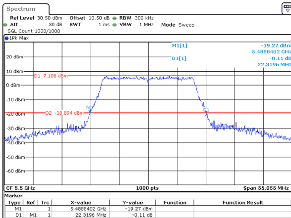
802.11ac20_5500MHz 22.320MHz
