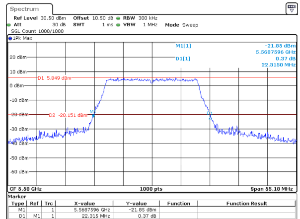
802.11ac20_5580MHz 22.315MHz
