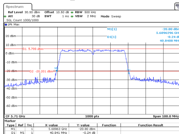
802.11ac40_5710MHz 40.841MHz
