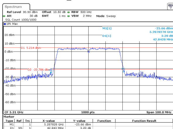
802.11ac40_5310MHz 42.843MHz
