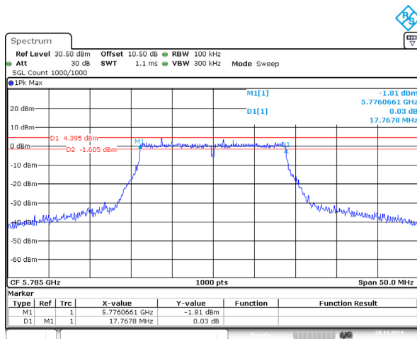
802.11ac20_5785MHz 17.768MHz
