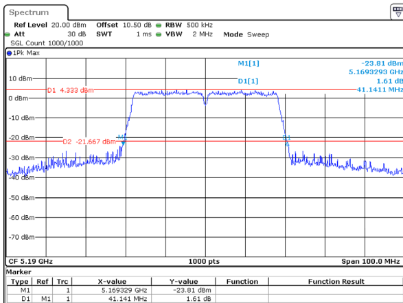
802.11ac40_5190MHz 41.141MHz
