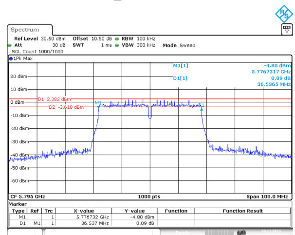
802.11ac40_5795MHz 36.537MHz
