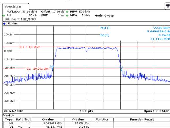
802.11ac40_5670MHz 41.141MHz
