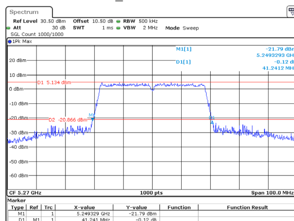
802.11ac40_5270MHz 41.241MHz
