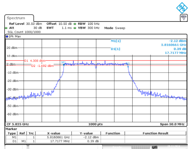
802.11ac20_5825MHz 17.718MHz
