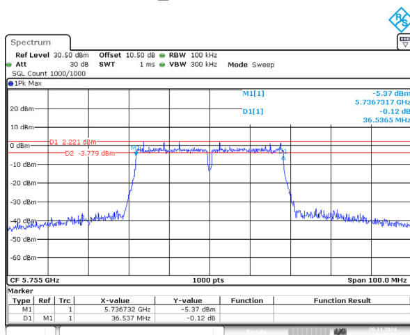
802.11ac40_5755MHz 36.537MHz
