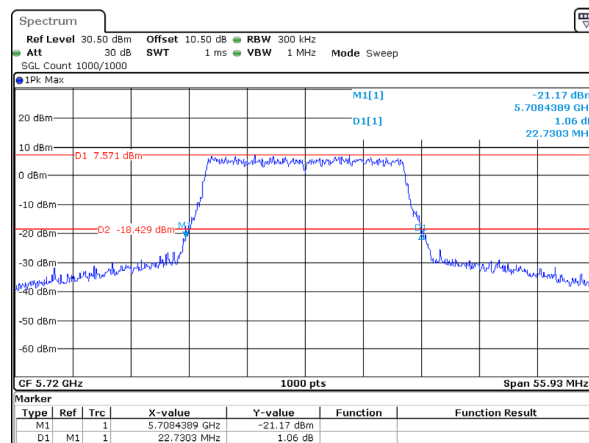
802.11ax20_5720MHz_RU_Full 22.730MHz
