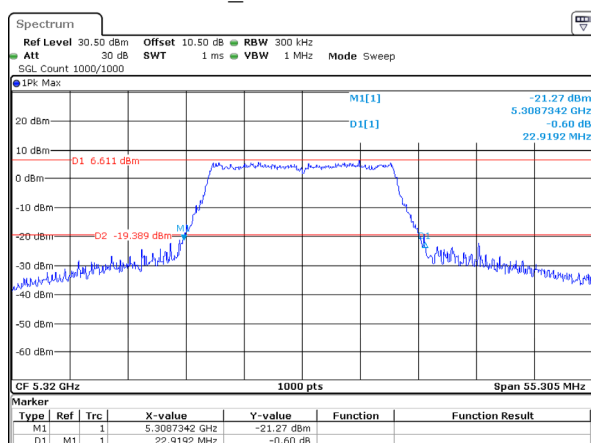
802.11ac20_5320MHz 22.919MHz
