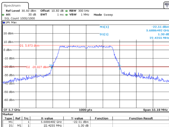
802.11ac20_5700MHz 22.426MHz
