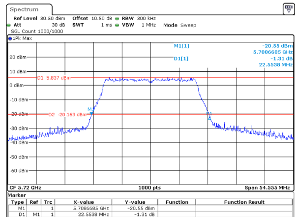
802.11ac20_5720MHz 22.554MHz
