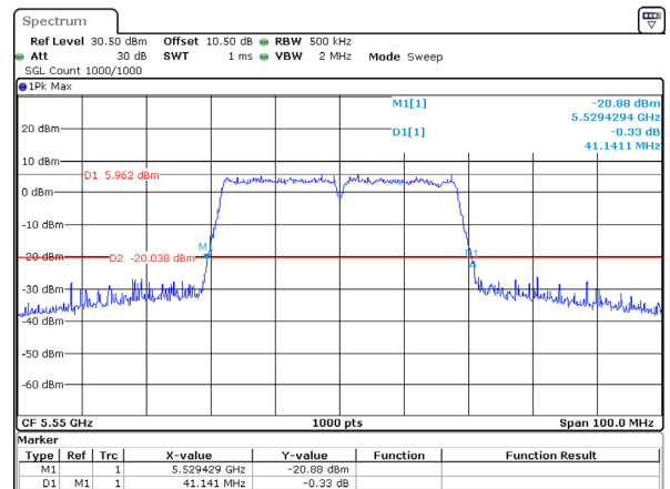
802.11ac40_5550MHz 41.141MHz
