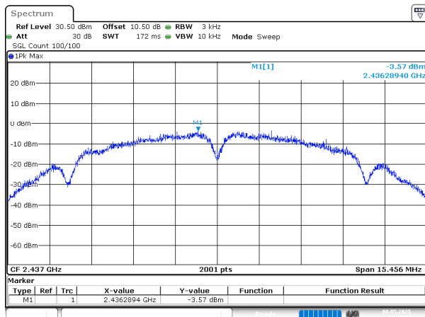
802.11b_2437MHz_Chain 1
